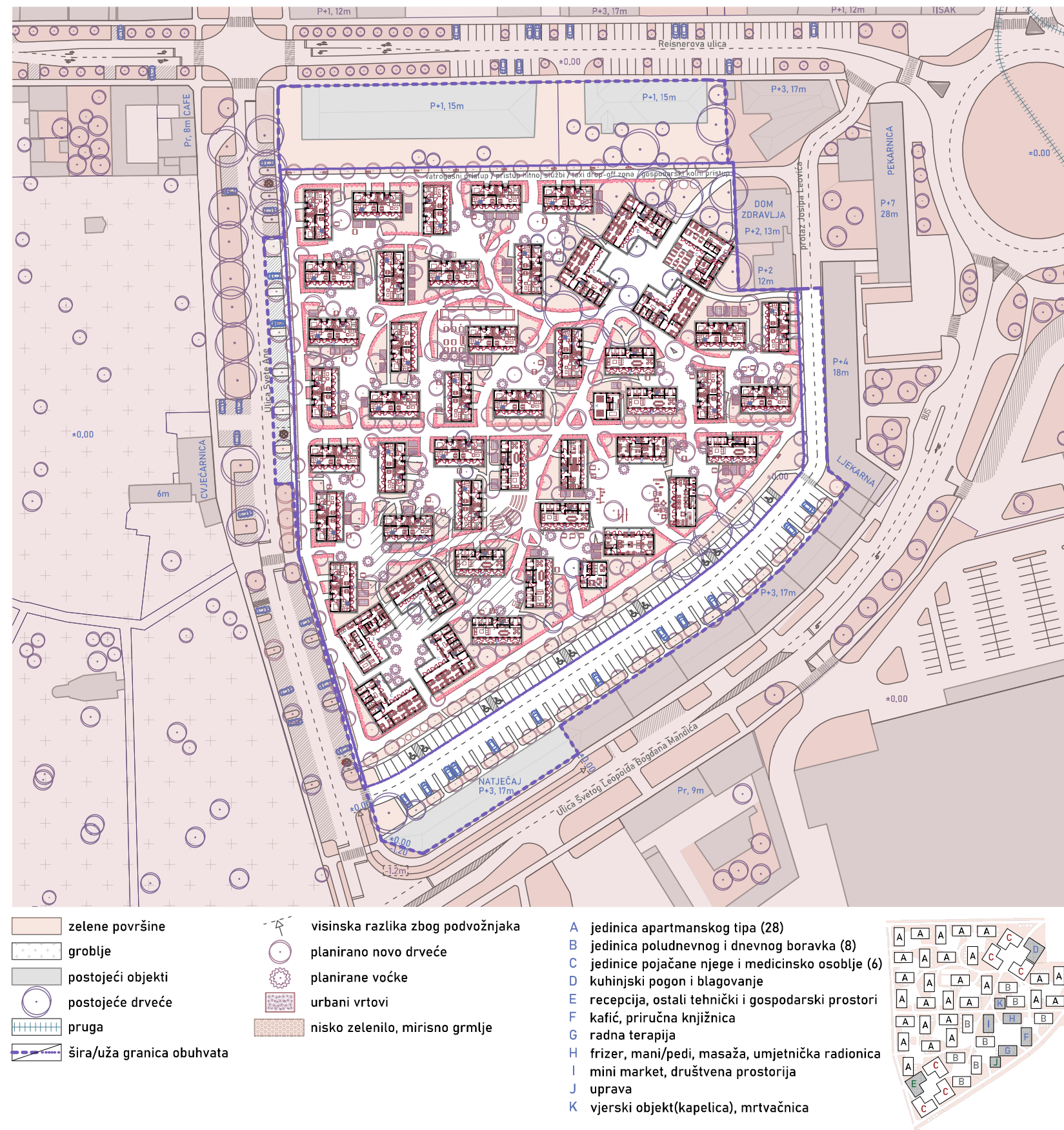
M 1:1500 SITUACIJSKI NACRT S TLOCRTOM PRIZEMLJA
