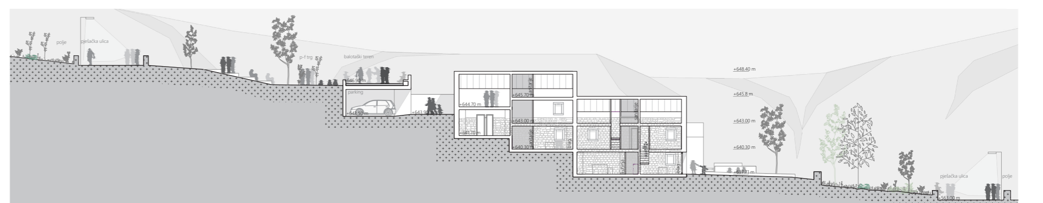
PRESJEK E-E
