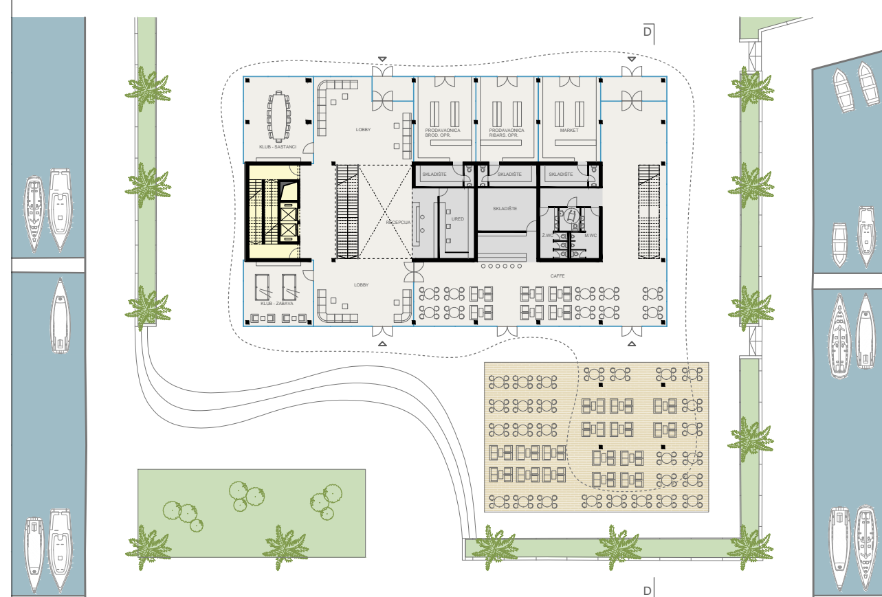
TLOCRT PRIZEMLJA
