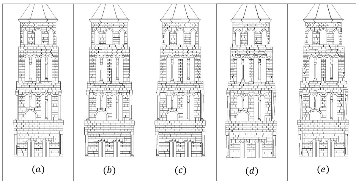
Slika 38. Nastanak i širenje pukotina po vremenskim koracima za Petrovac, a_g=0.22\text{ m/s}^2 : a) t=12.5\text{ s} ; b) t=13.5\text{ s} ; c) t=15\text{ s} ; d) t=25\text{ s} ; e) t=51.2\text{ s}
