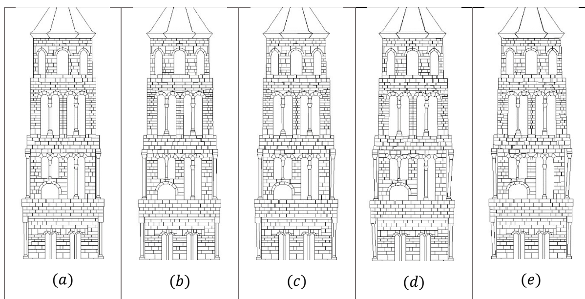
Slika 38. Nastanak i širenje pukotina po vremenskim koracima za Petrovac, a_g=0.22 m/s 2 : a) t=12.5 s; b) t=13.5 s; c) t=15 s; d) 25 s; e) t=51.2 s
