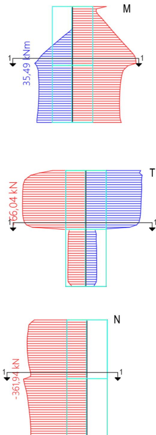
Slika 8.52. Prikaz rezultata u zidu B1
