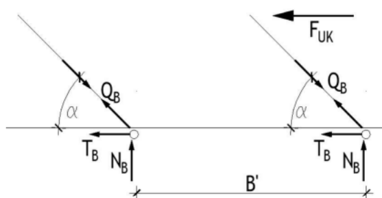
Slika 2.10. Shematski prikaz djelovanja sila za kombinaciju 2
