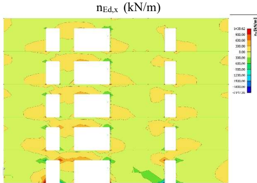
C3x) Proračunske vlačne sile za ANV 1:
