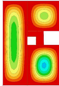
Progibi ploča. U_z (mm) – GSU – 1 ( \delta_{\max,d} \leq L/1000 )
