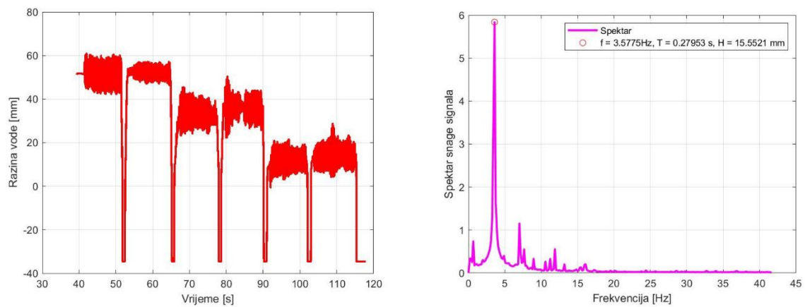
Slika 3.14 Eksperiment 3 T_{motora}=0.25
