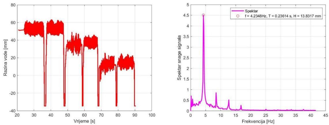
Slika 3.13 Eksperiment 2 T_{motora}=0.2
