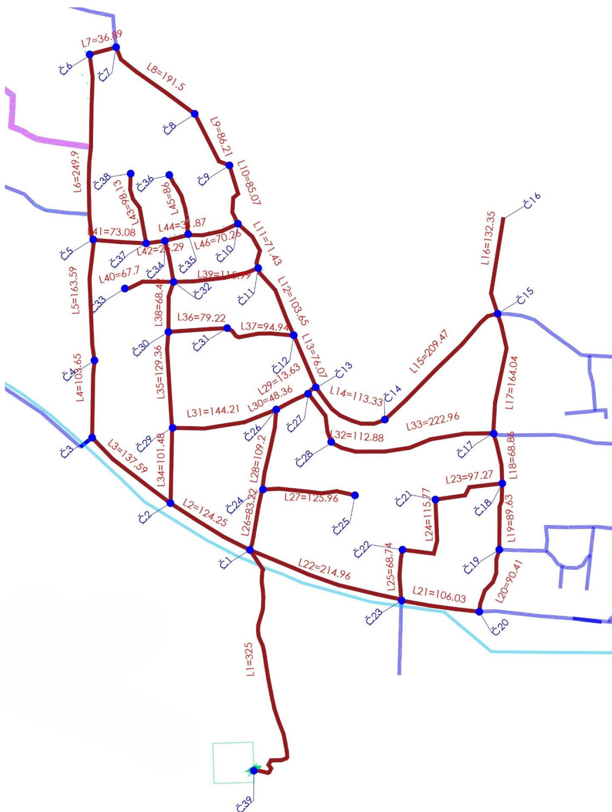
Slika 3. Izdvojeni dio vodovodne mreže naselja Preko za hidraulički proračun
