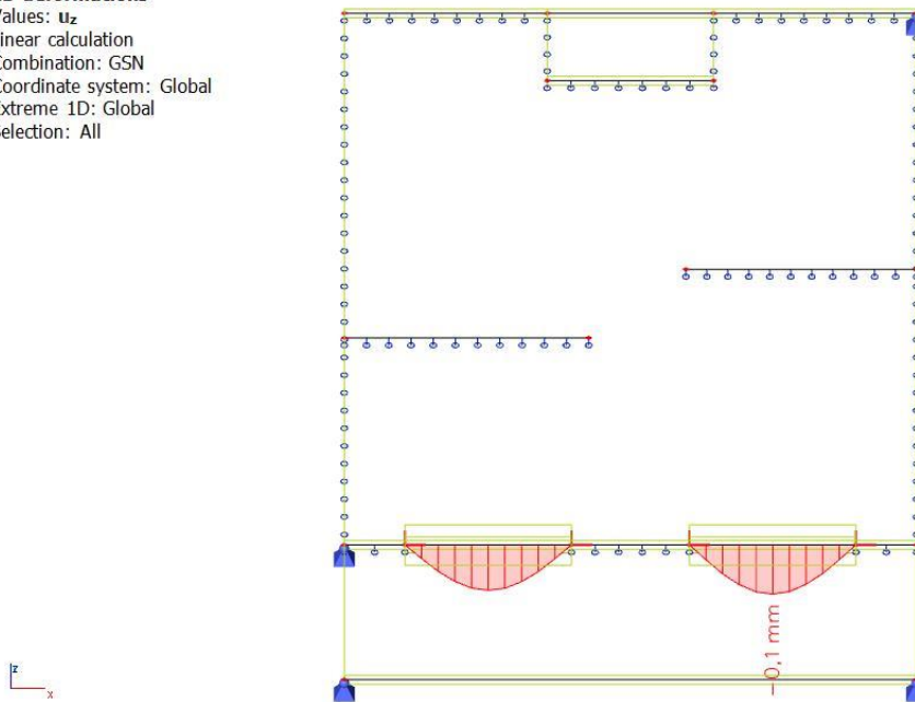
Slika 4.27. Progib za q_{sda} = 1.35G + 1.5Q
