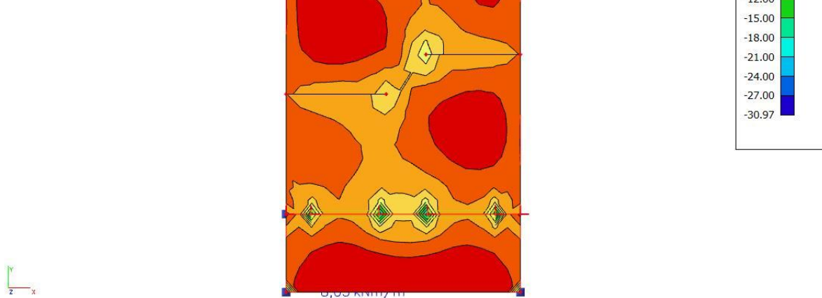
Slika 4.6. M_{Sd,x} ( kN/m^2 ) = računski momenti savijanja u smjeru lokalnih osi za q_{sd} = 1.0G+1.0Q
