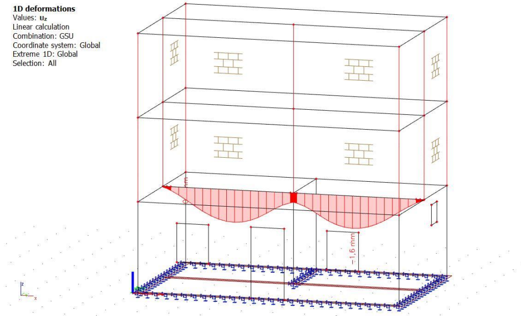
Slika 4.47. Progib za q_{sd} = 1.35G + 1.5Q
