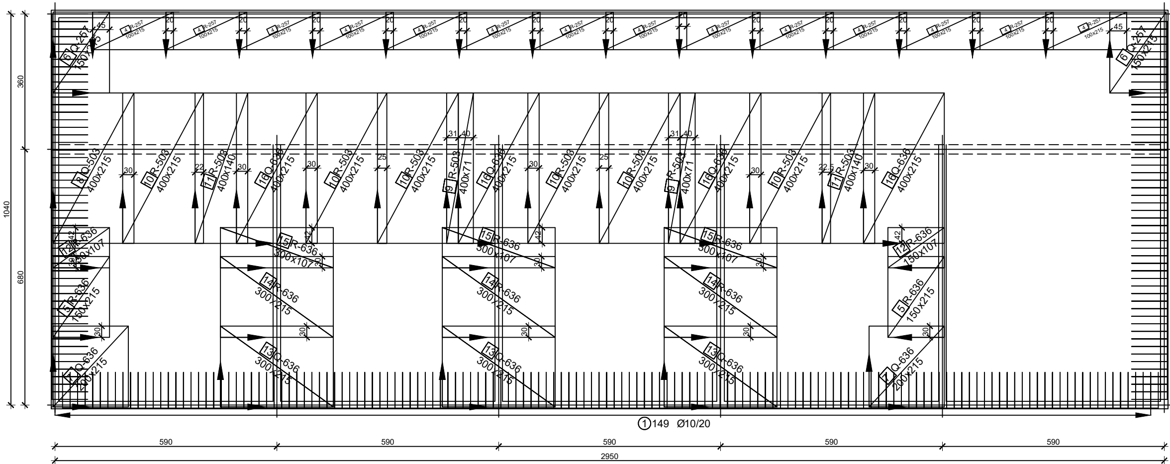
Armatura ploče pozicija 400 - gornja zona zona 1:100
