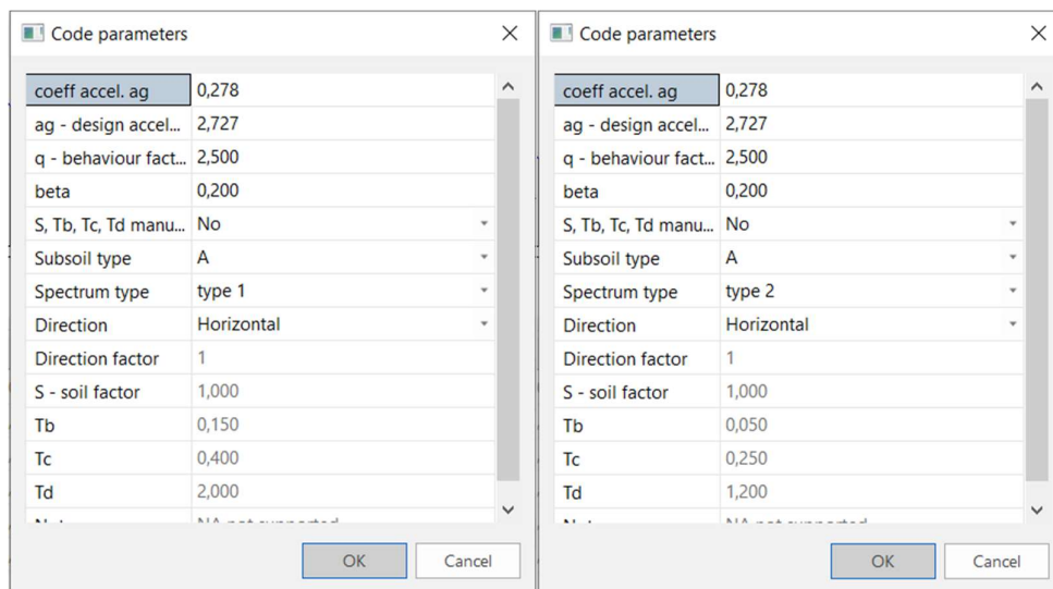
Slika 23. Karakteristike seizmičkog opterećenja
