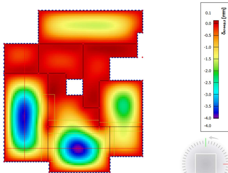
Dijagram 46. Prikaz deformacija za stvarnu armaturu u ploči (Q503)
