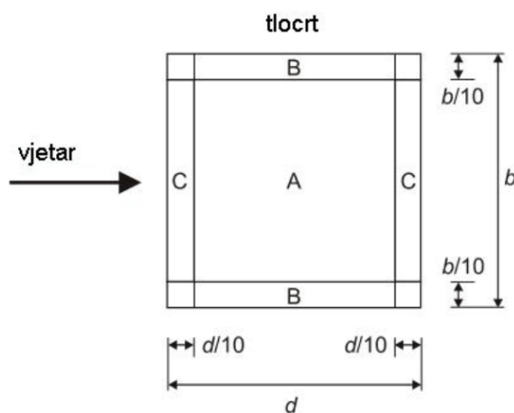
Slika 4.4. Zone djelovanja vjetra na nadstrešnicu
