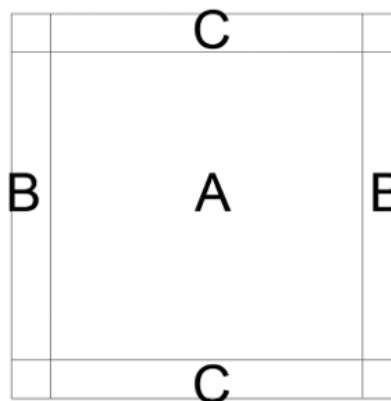
Slika 4.6. Zone djelovanja vjetra na nadstrešnicu (Y-smjer)
