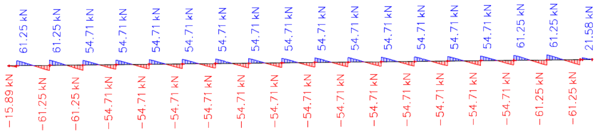
Slika 9.14. Dijagram poprečnih sila ( V_z )
