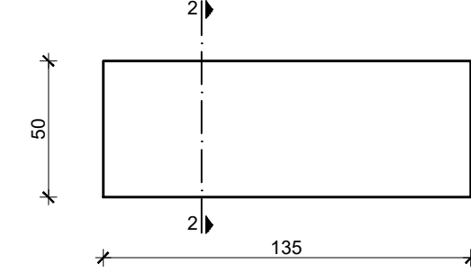
Tlocrt
