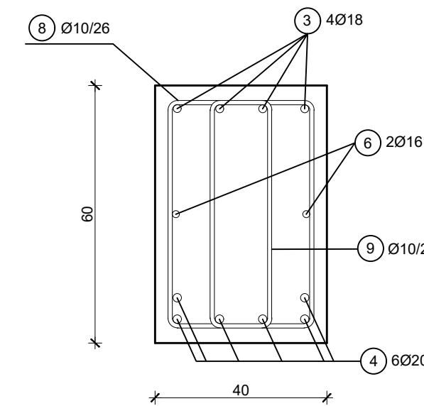
PRESJEK 3-3 MJ 1:12.5
