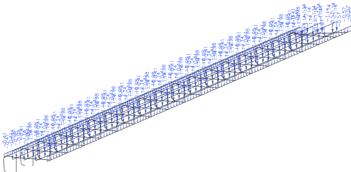
Slika 9.3. Opterećenje snijegom
