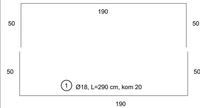
Tlocrt - donja zona
