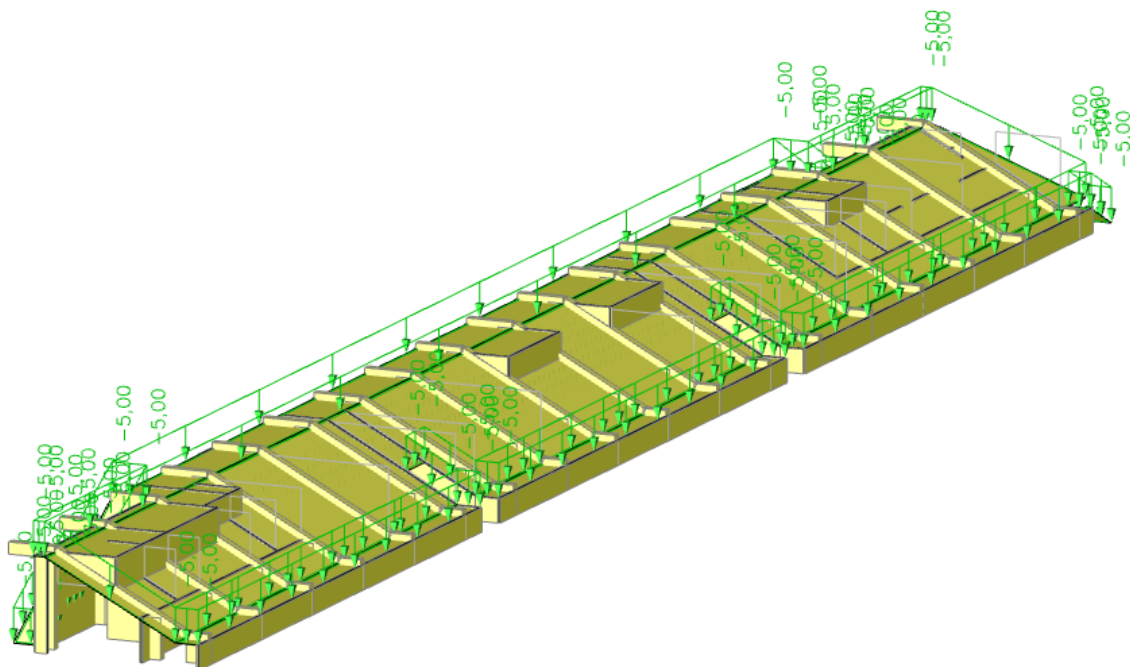
Slika 10.3. Pokretno opterećenje
