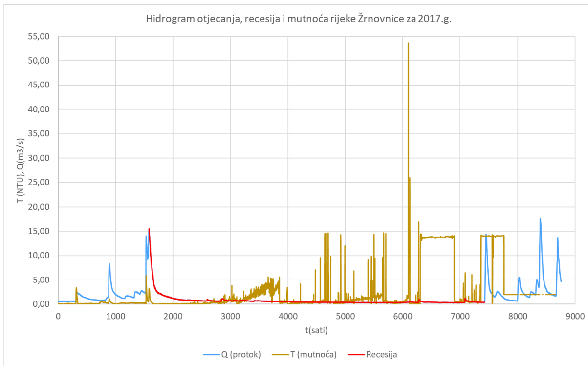
Slika 46. Hidrogram otjecanja, recesija i mutnoća rijeke Žrnovnice za 2017. godinu
