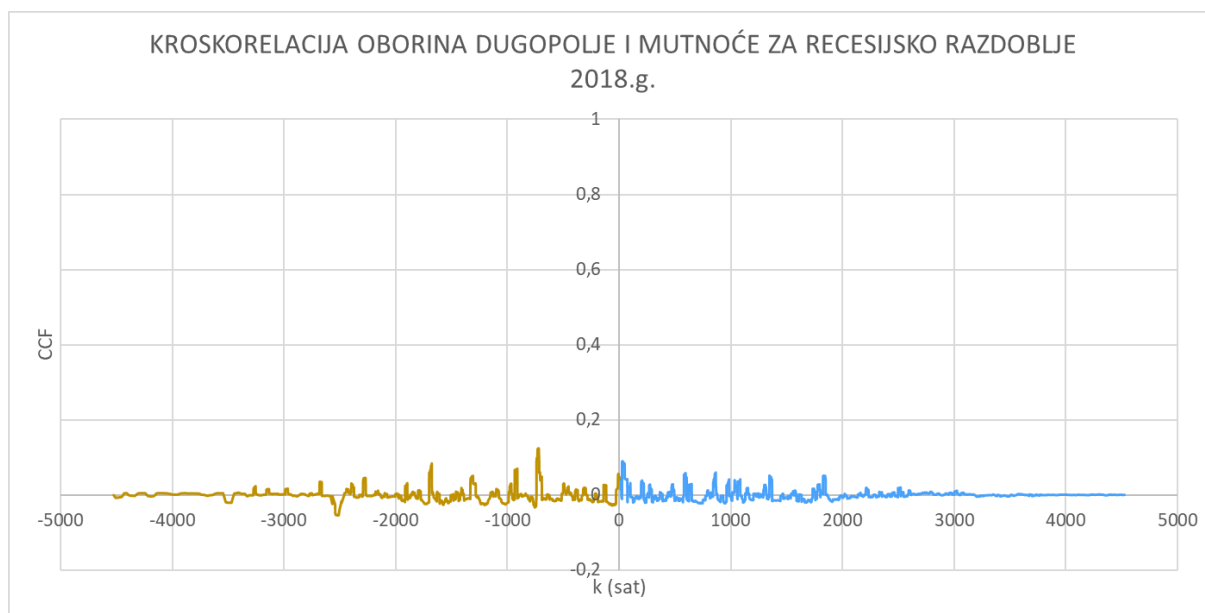
Slika 105. Kroskorelacija oborina Dugopolje i mutnoće za recesijsko razdoblje 2018.
