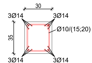
PRESJEK 1-1
