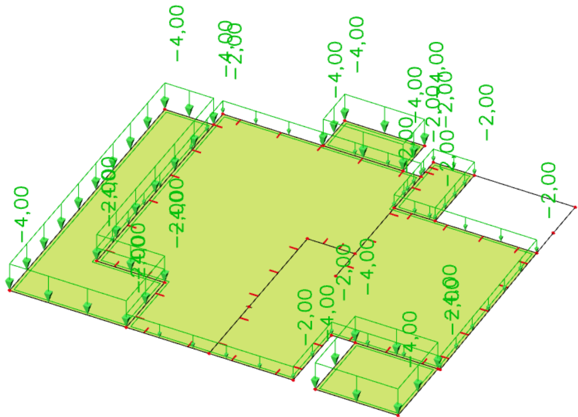
Slika 7.21. Promjenjivo opterećenje (korisno) q=2,0 , za balkone q=4,0 ( \text{kN/m}^2 )
