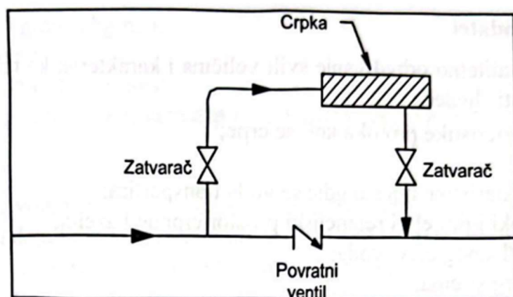
Shema izvedbe
