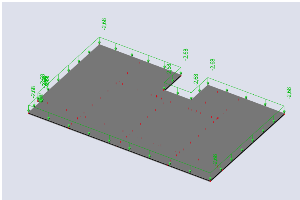
Slika 7 Dodatno stalno djelovanje G_1 [kN/m 2 ]
