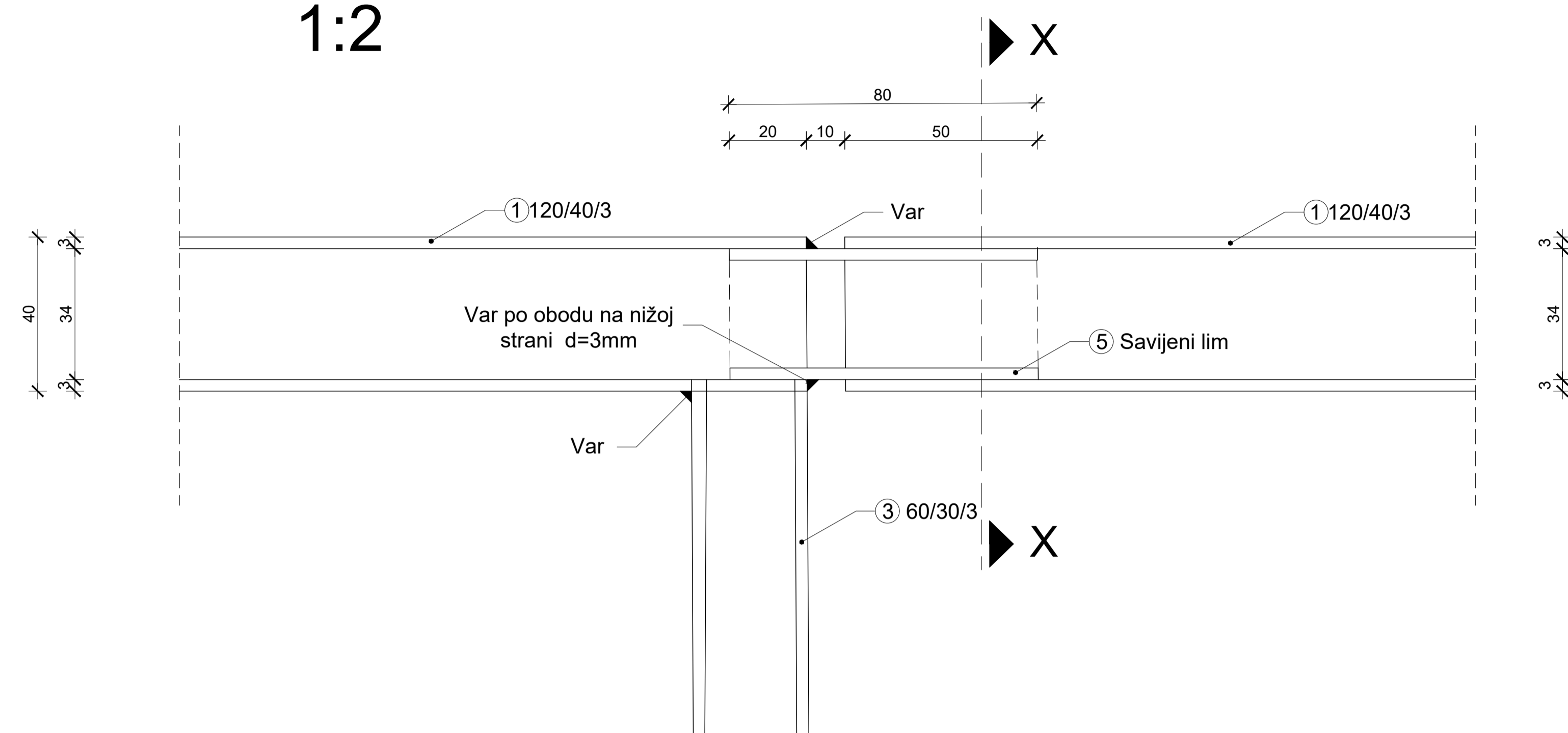
Detalj D 2 1:2
