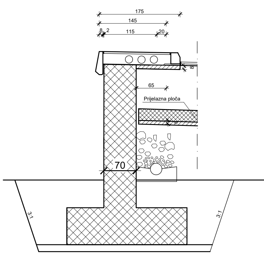
Presjek 7-7
