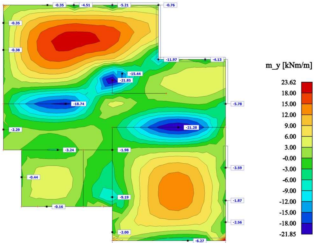
Moment m_y
