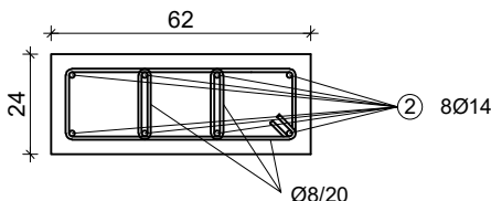
DETALJ ⑩
