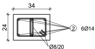
DETALJ ⑨
