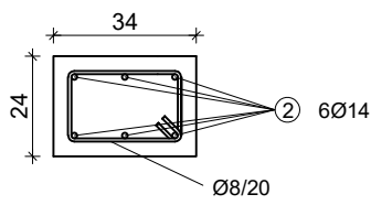
DETALJ ⑤
