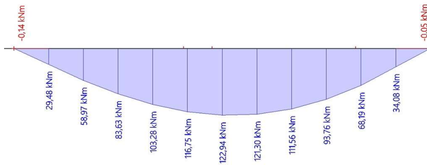
Moment M_y
