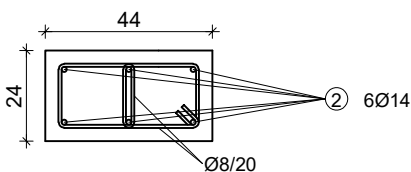
DETALJ ⑩
