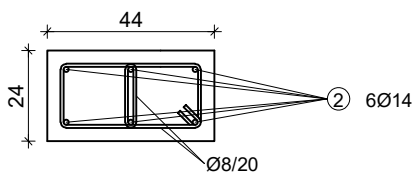
DETALJ ⑩
