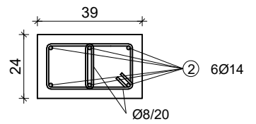
DETALJ ⑧
