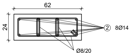
DETALJ ⑩
