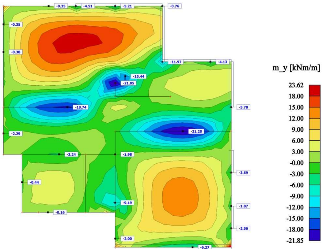
Moment m_y
