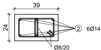
DETALJ ⑧
