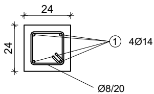
DETALJ ⑨
