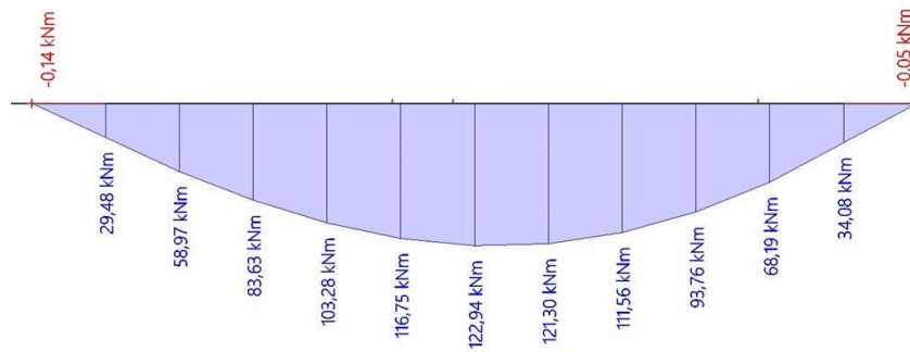
Moment M_y
