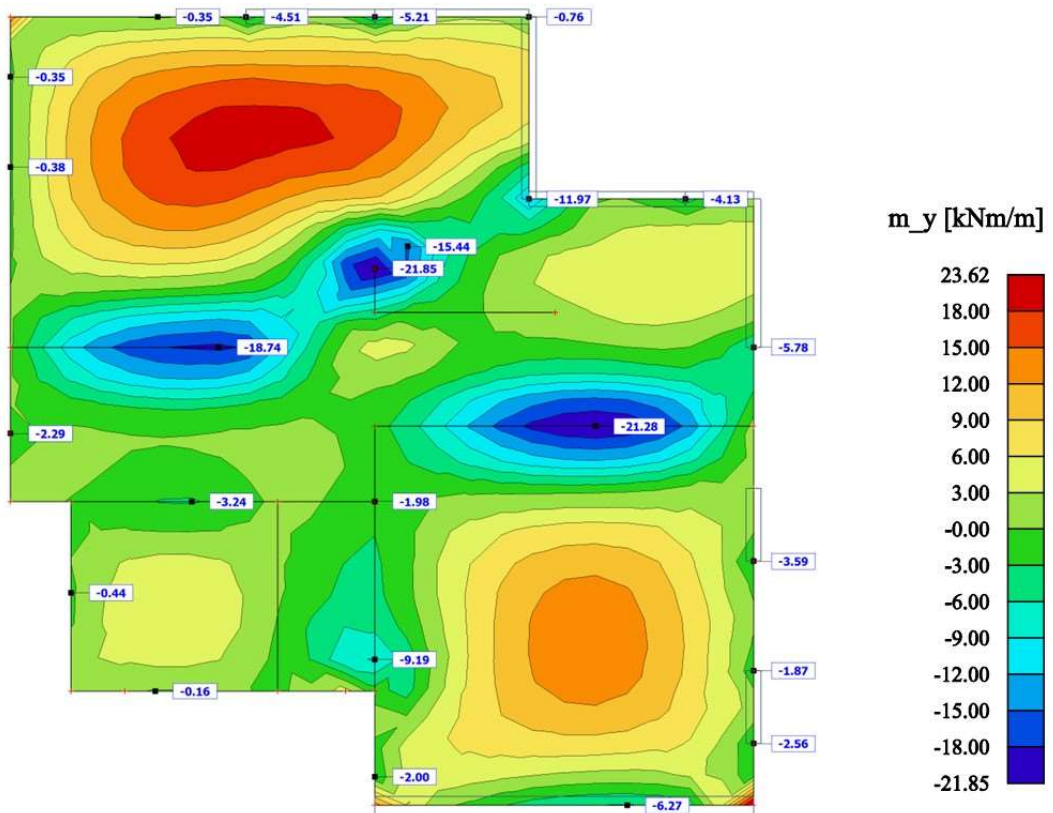
Moment m_y
