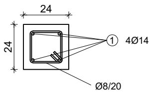
DETALJ ⑨
