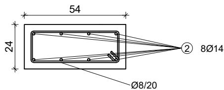
DETALJ ⑤
