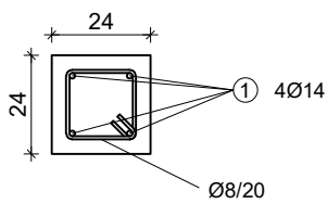
DETALJ ④
