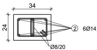
DETALJ ⑨
