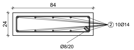
DETALJ ③
