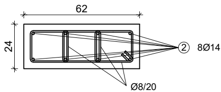
DETALJ ⑩
