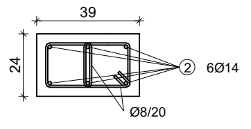
DETALJ ⑧
