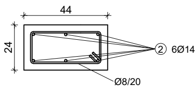
DETALJ ④
