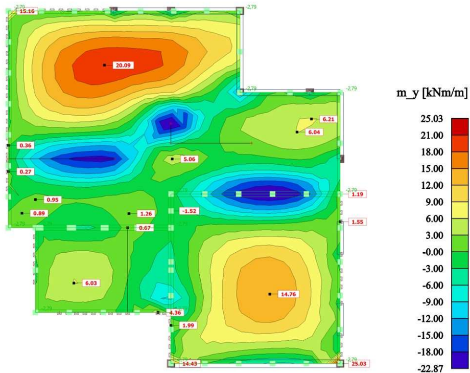
Moment m_y
