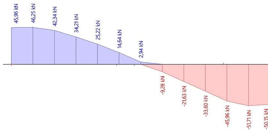
Poprečna sila V
