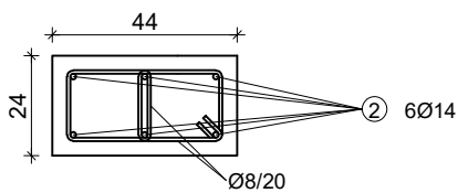
DETALJ ⑩
