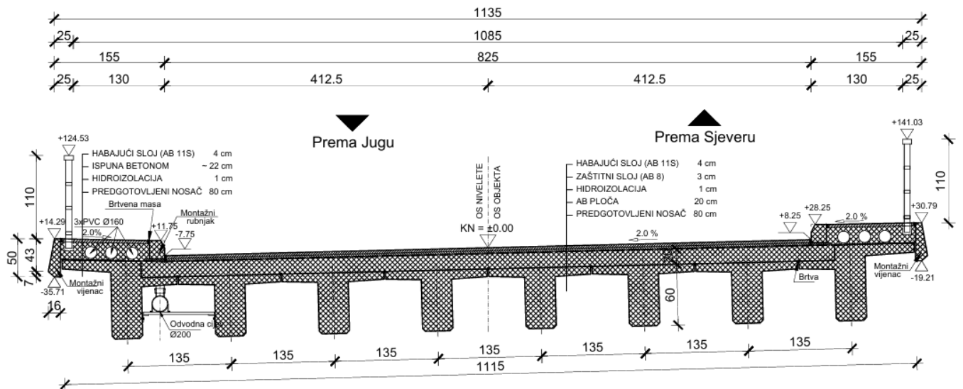
Slika 1: Poprečni presjek rasponske konstrukcije
