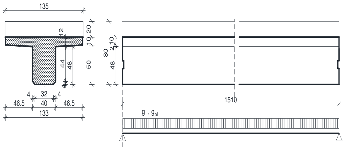
Slika 2: Uzdužna i poprečna dispozicija jednog nosača
