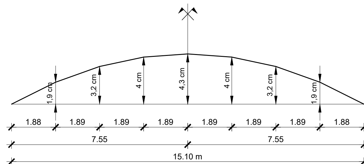
Shema nadvišenja
