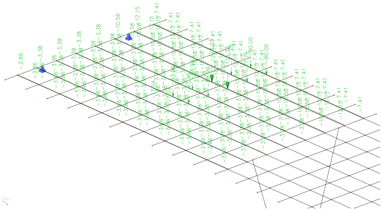
Slika 15: Pokretno opterećenje za maksimalni moment u polju
