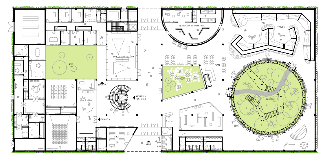
TLOCRT PRIZEMLJA
