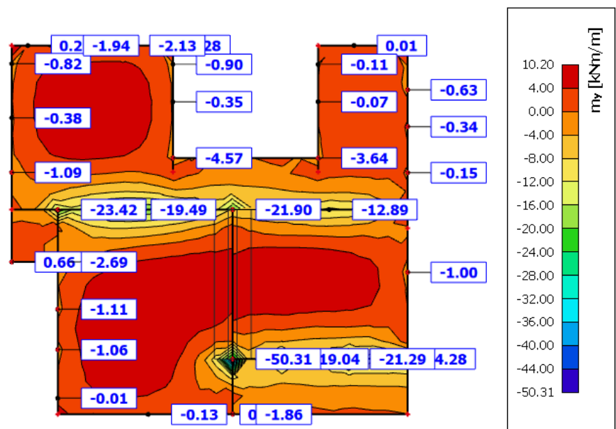
Moment m_y
