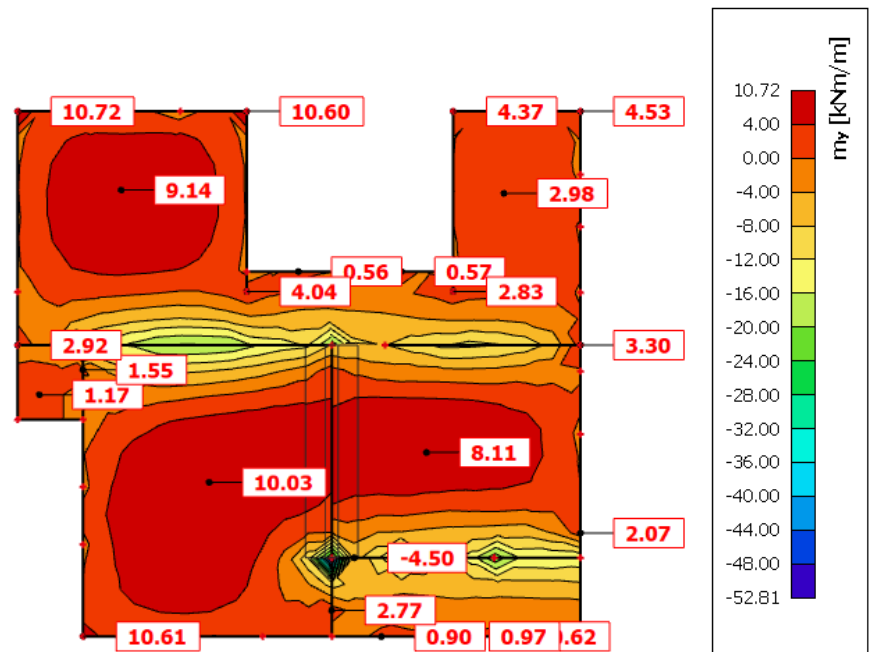
Moment m_y
