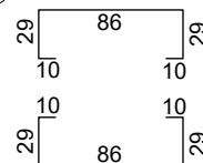
⑤ 2 \phi 12 L=164
