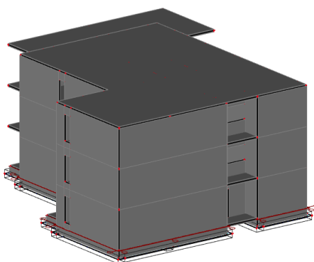
Slika 2.2 Proračunski model objekta – pogled 2
