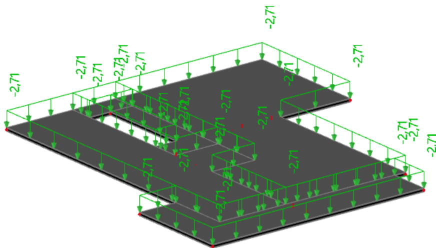
Slika 5.2.1 Dodatno stalno djelovanje G1 [kN/m 2 ]
