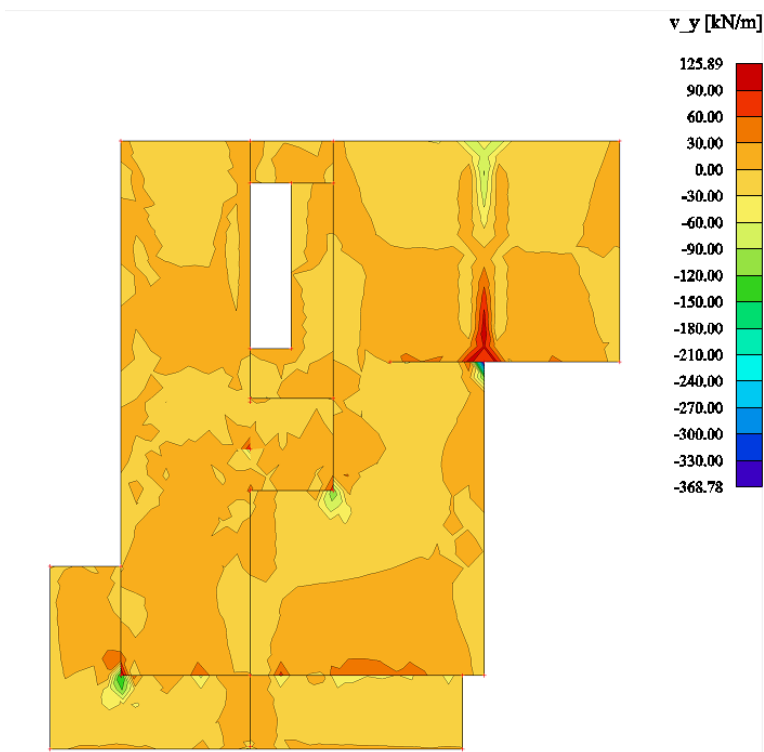
Slika 7.6 Poprečne sile V_{Ed,y} (kN/m) za GSN-1
