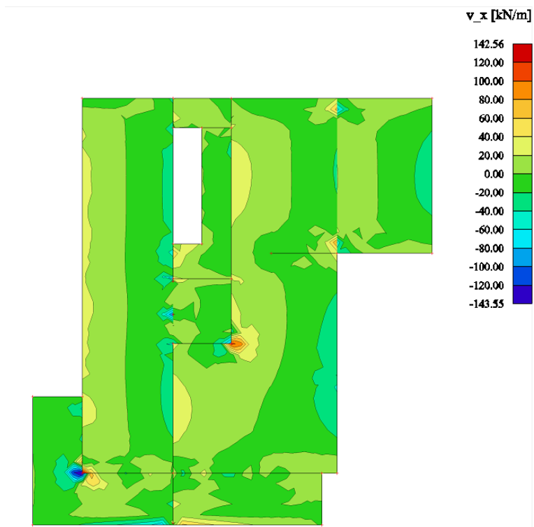
Slika 7.5 Poprečne sile V_{Ed,x} (kN/m) za GSN-1
