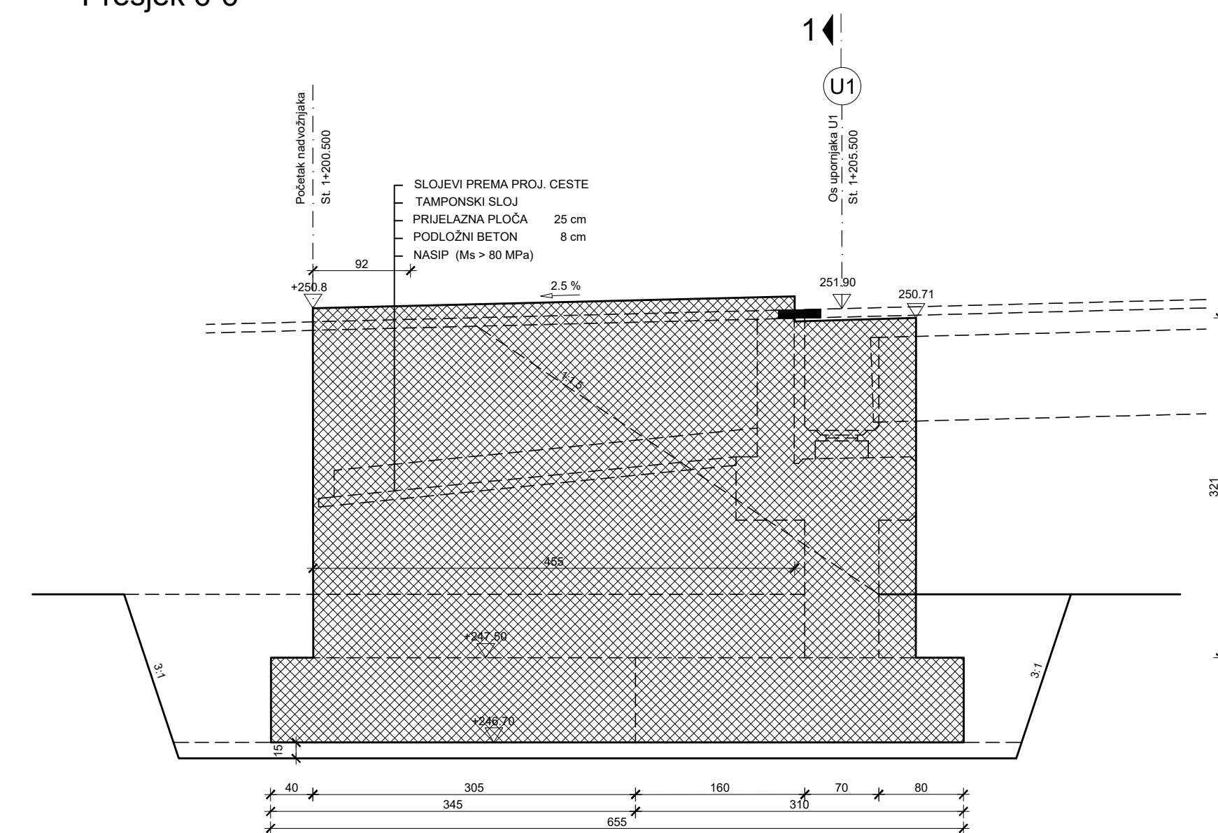
Presjek 6-6
