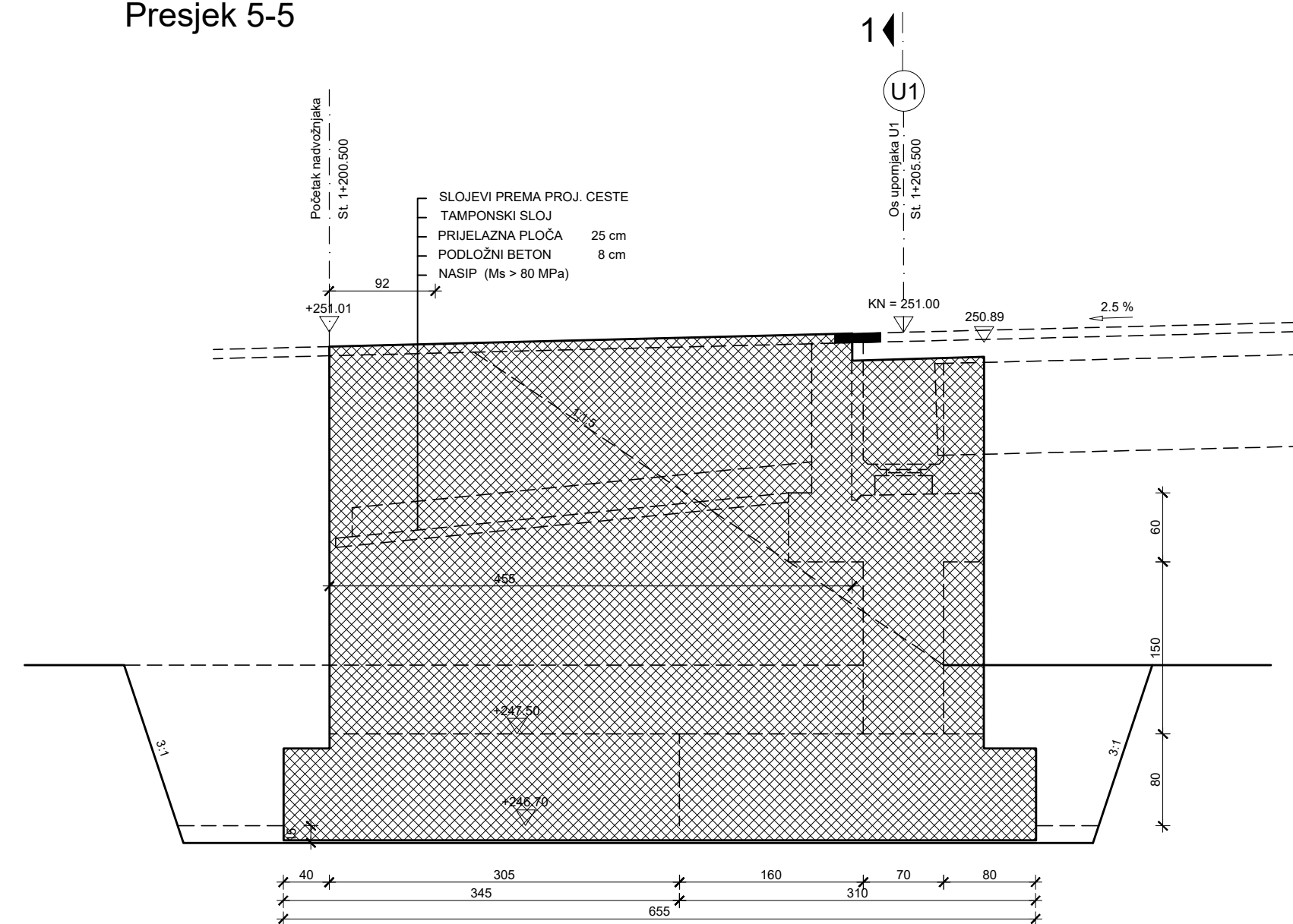
Presjek 5-5
