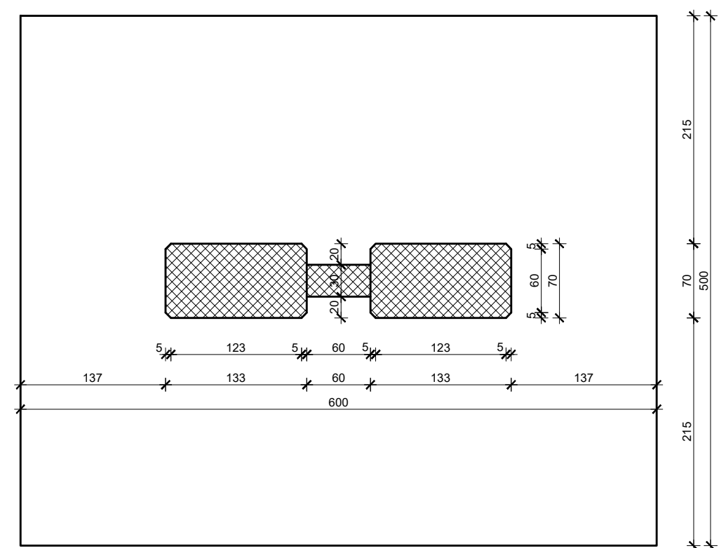
Presjek 4-4
