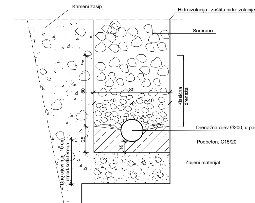
Detalj drenaze
