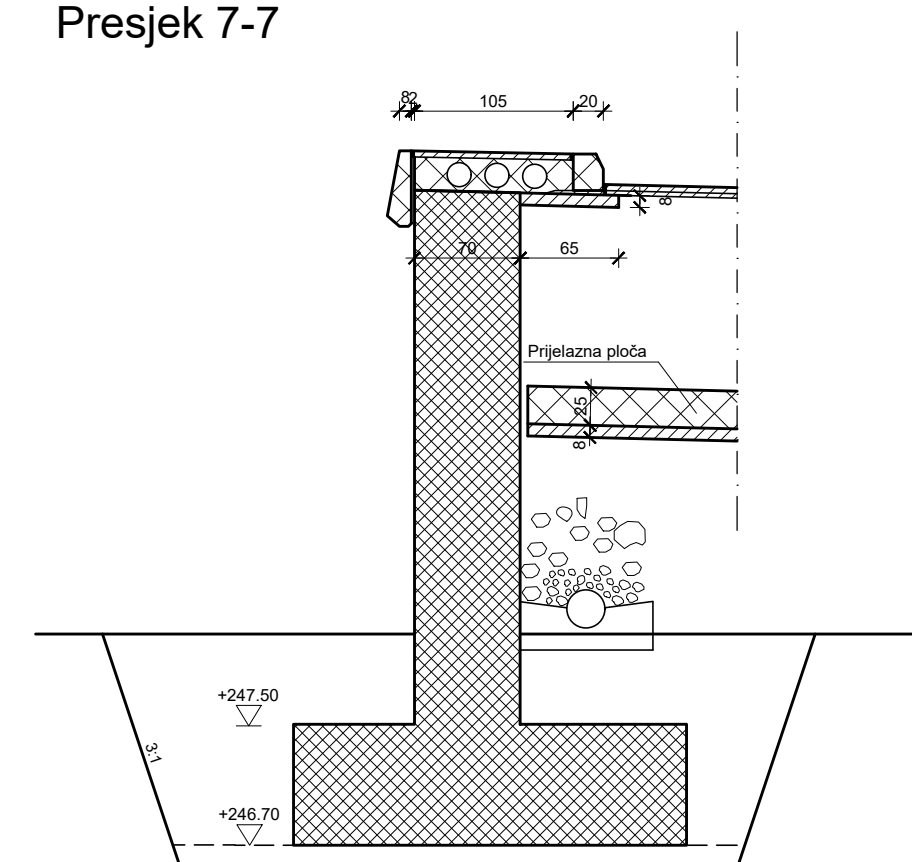
Presjek 7-7
