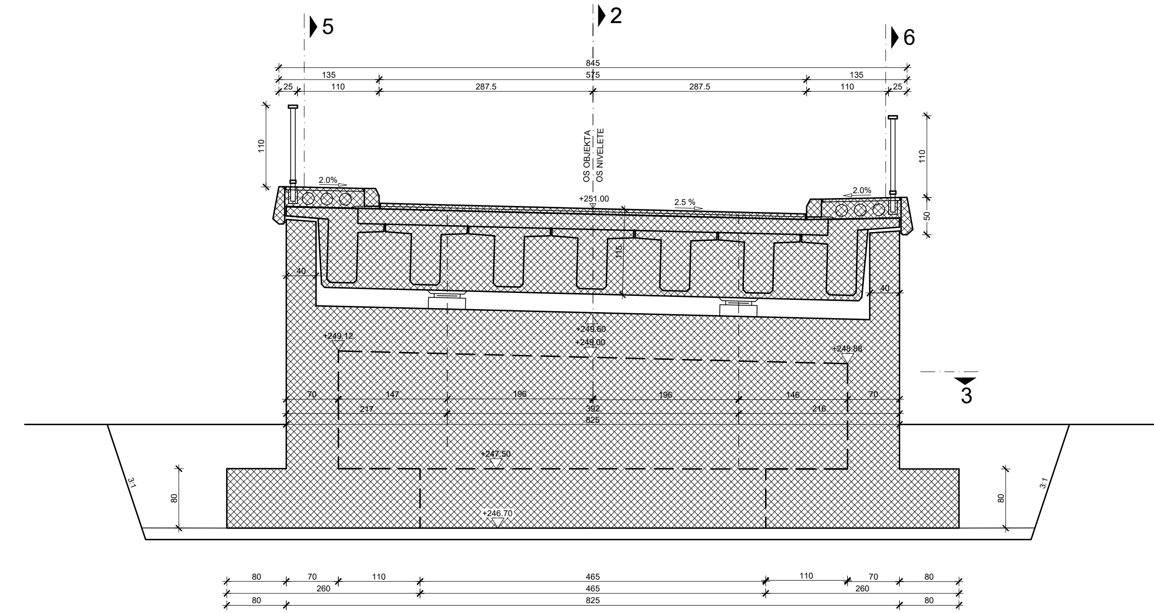
Presjek 1-1
