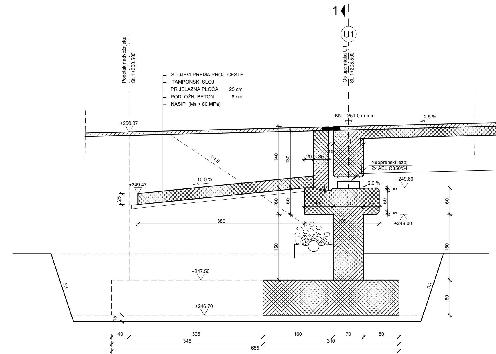
Presjek 2-2
