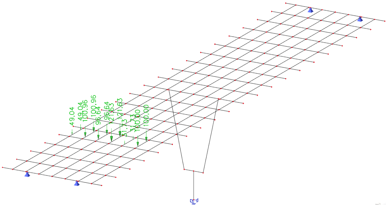
Slika 20: Prikaz tipskog vozila za maksimalni moment savijanja pri stupu
