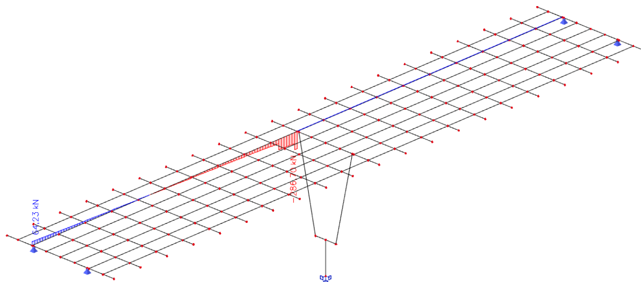
Slika 30: Pokretno opterećenje – maksimalna poprečna sila pri stupu – poprečne sile ( V_z ) u kN
