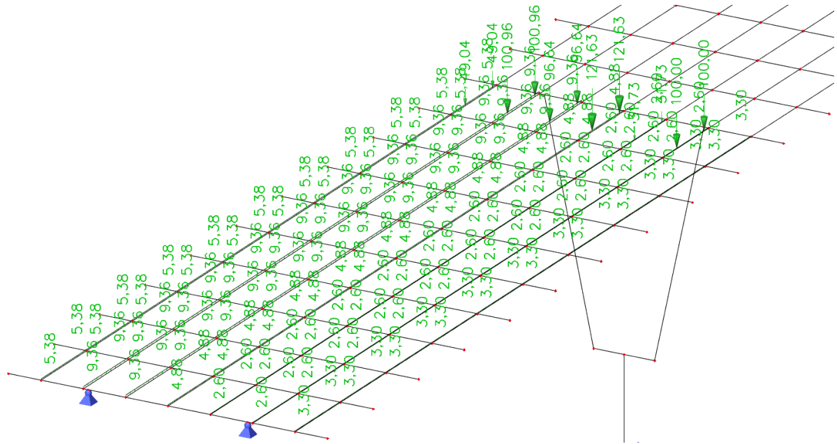
Slika 27: Pokretno opterećenje za maksimalnu poprečnu silu pri stupu
