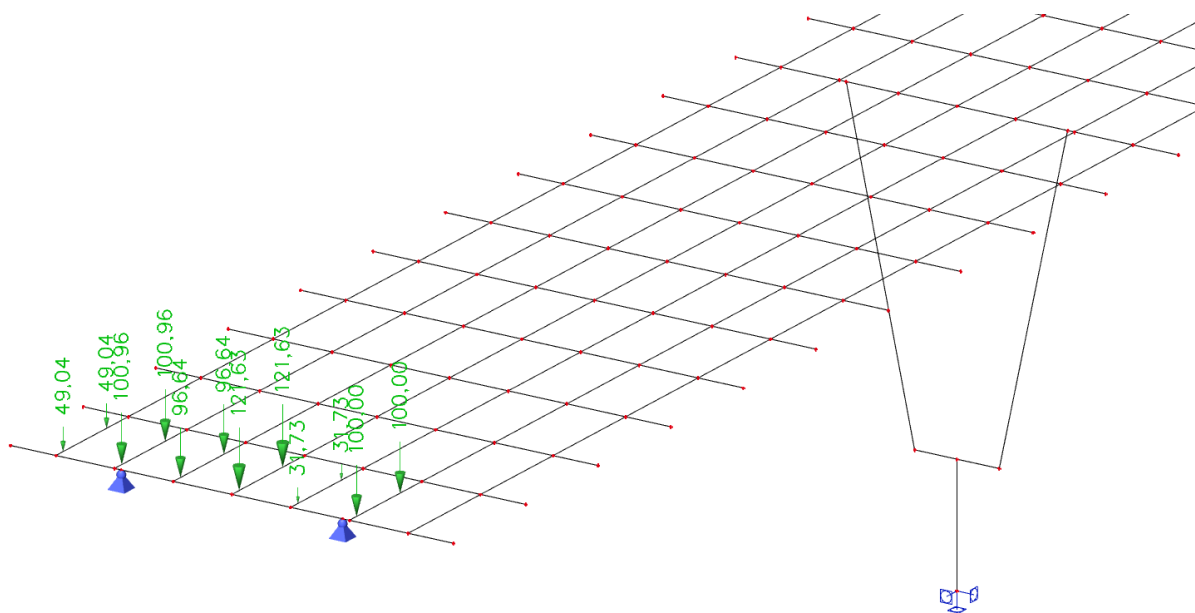
Slika 24: Prikaz tipskog vozila za maksimalnu poprečnu silu pri upornjaku
