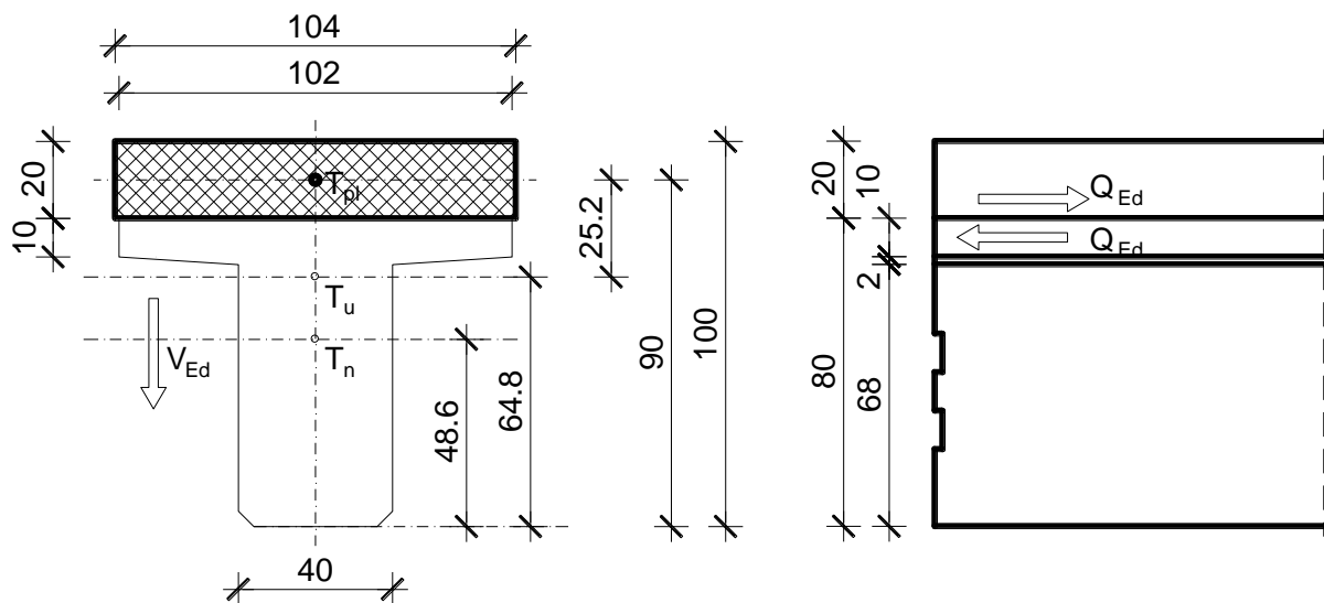
Slika 32: Poprečni presjek spregnutog T nosača
