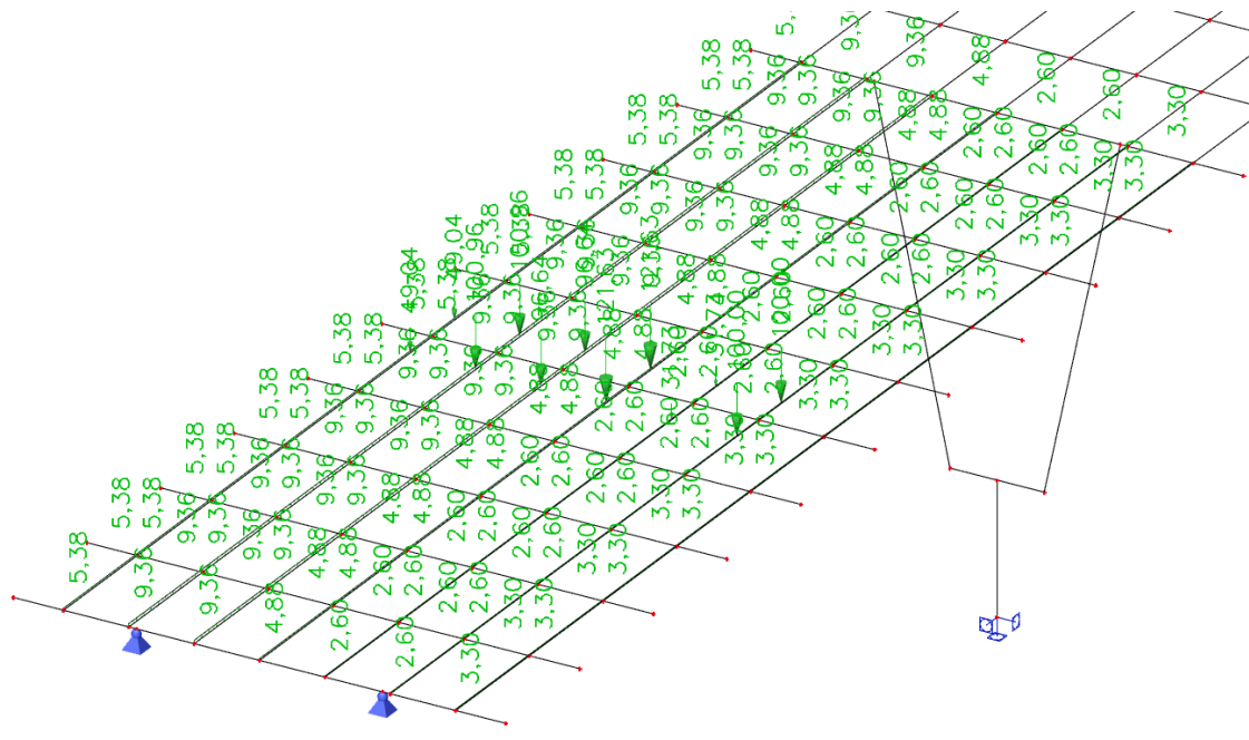
Slika 15: Pokretno opterećenje za maksimalni moment savijanja u polju
