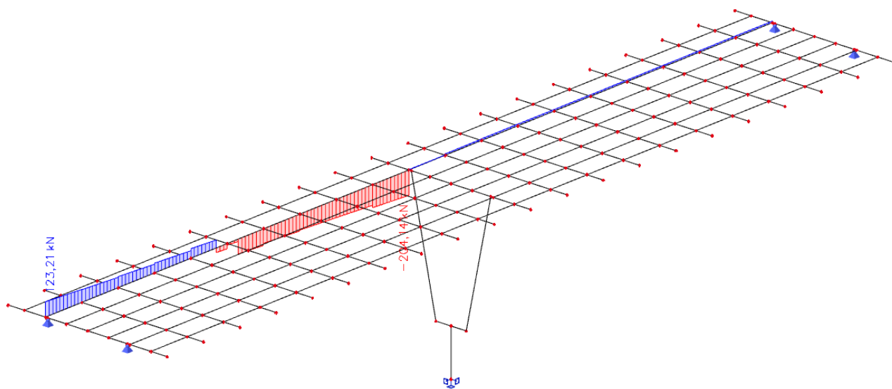
Slika 18: Pokretno opterećenje – maksimalni moment savijanja u prvom polju – poprečne sile ( V_z ) u kN
