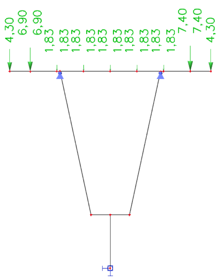
Slika 10 i 11: Dodatno stalno opterećenje
