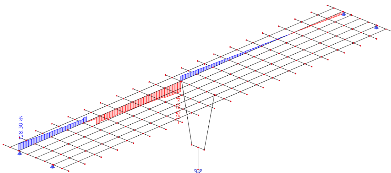
Slika 22 Pokretno opterećenje – maksimalni moment savijanja pri stupu – poprečne sile ( V_z ) u kN:
