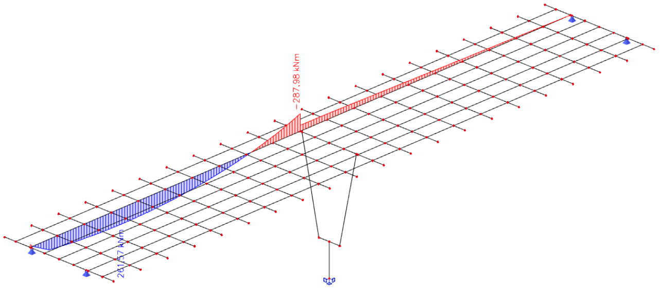
Slika 25: Pokretno opterećenje – maksimalna poprečna sila pri upornjaku – momenti savijanja ( M_y ) u kNm
