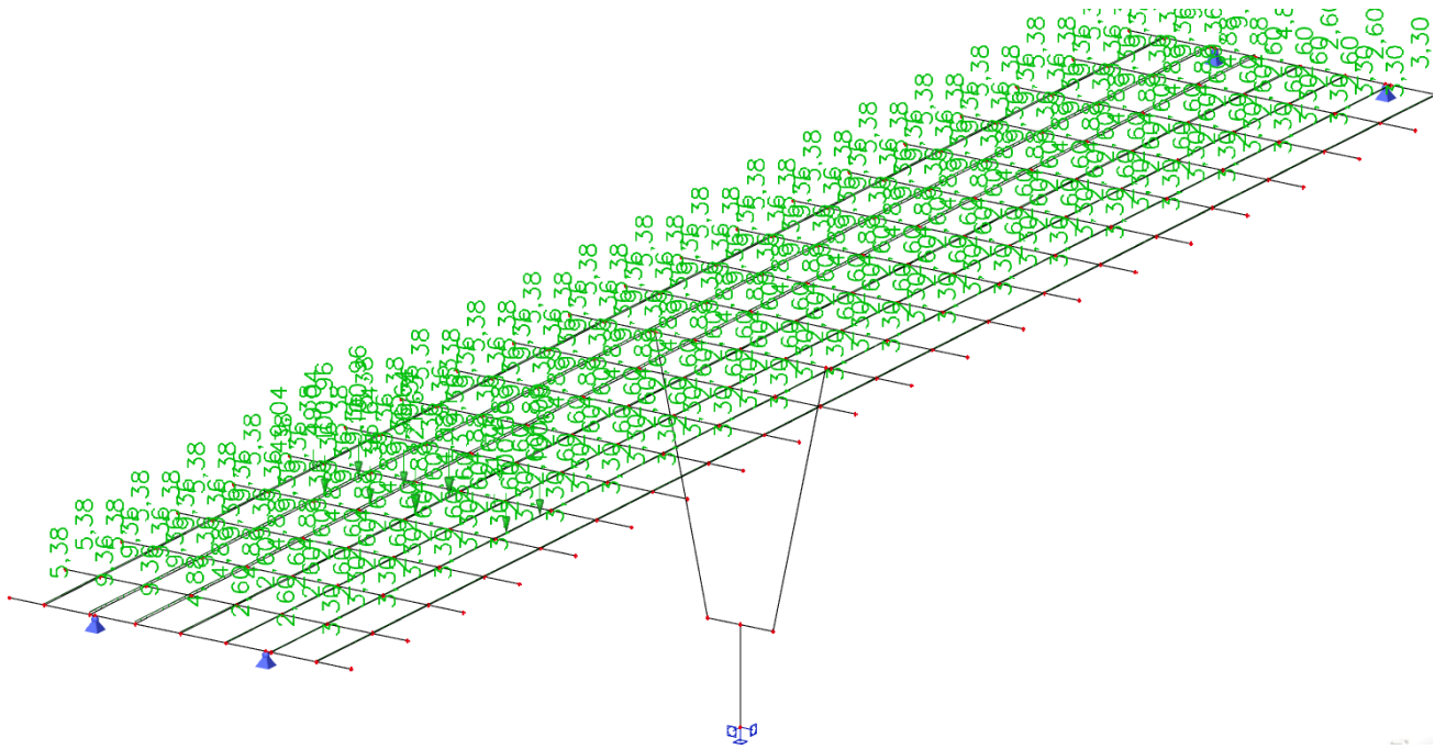
Slika 19: Pokretno opterećenje za maksimalni moment savijanja pri stupu
