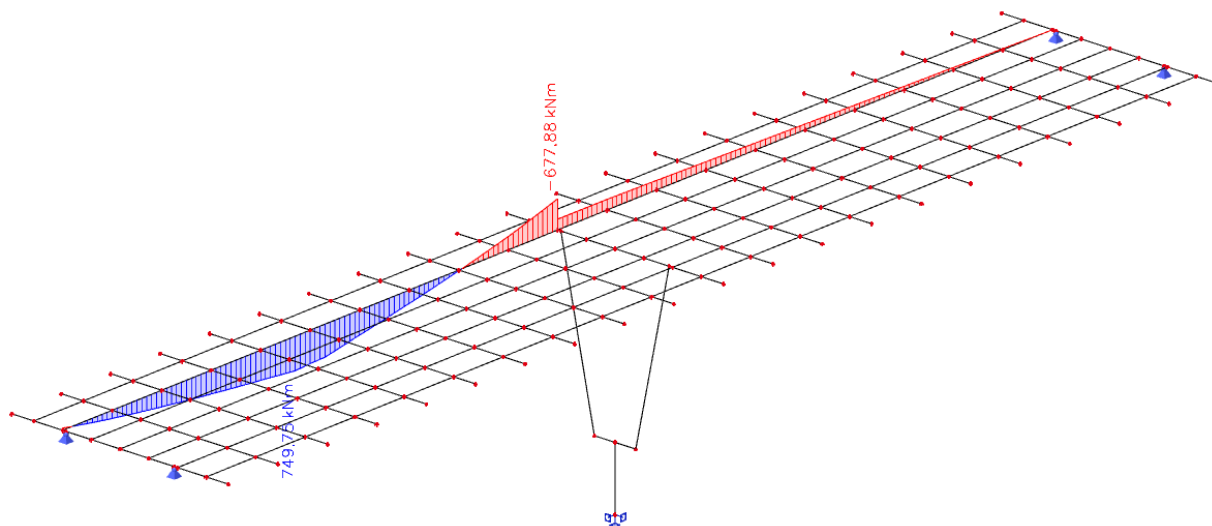
Slika 17: Pokretno opterećenje – maksimalni moment savijanja u prvom polju – momenti savijanja ( M_y ) u kNm
