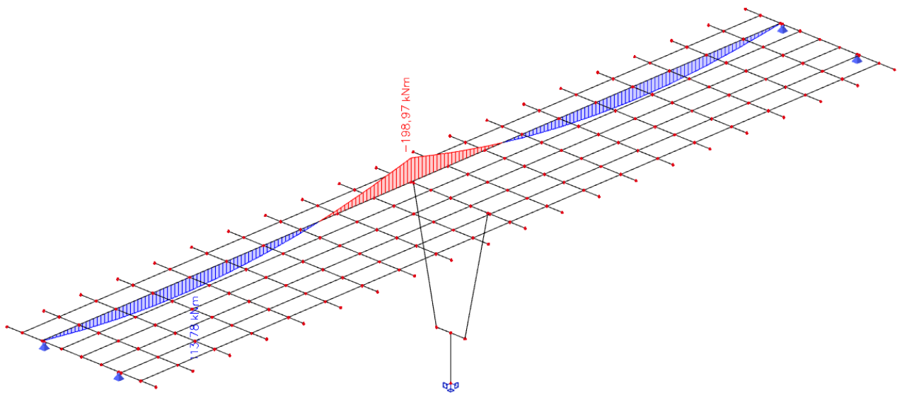
Slika 12: Dodatno stalno opterećenje – momenti savijanja ( M_y ) u kNm
