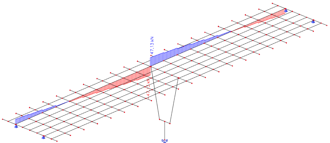
Slika 12: Dodatno stalno opterećenje – poprečna sila ( V_z ) u kN
