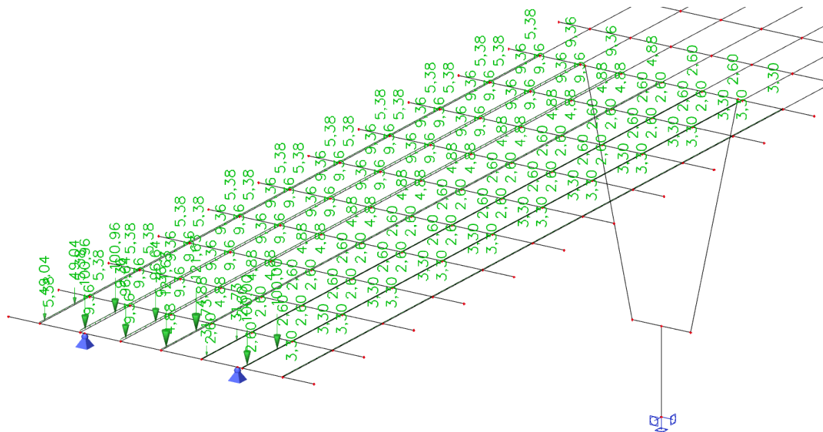
Slika 23: Pokretno opterećenje za maksimalnu poprečnu silu pri upornjaku
