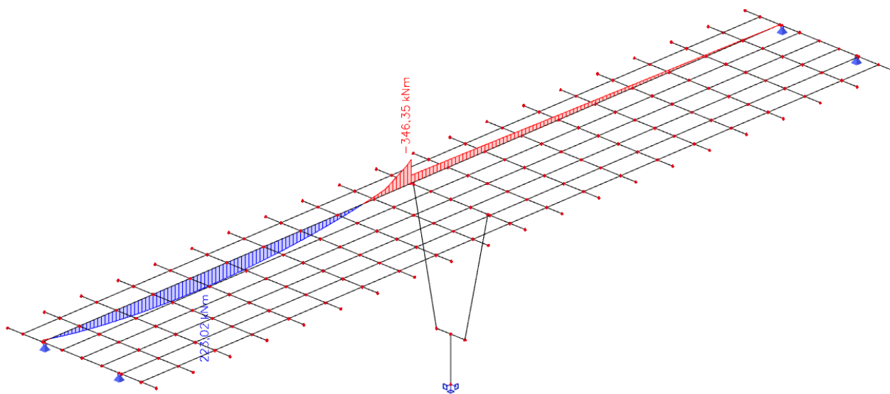
Slika 29: Pokretno opterećenje – maksimalna poprečna sila pri stupu – momenti savijanja ( M_y ) u kNm
