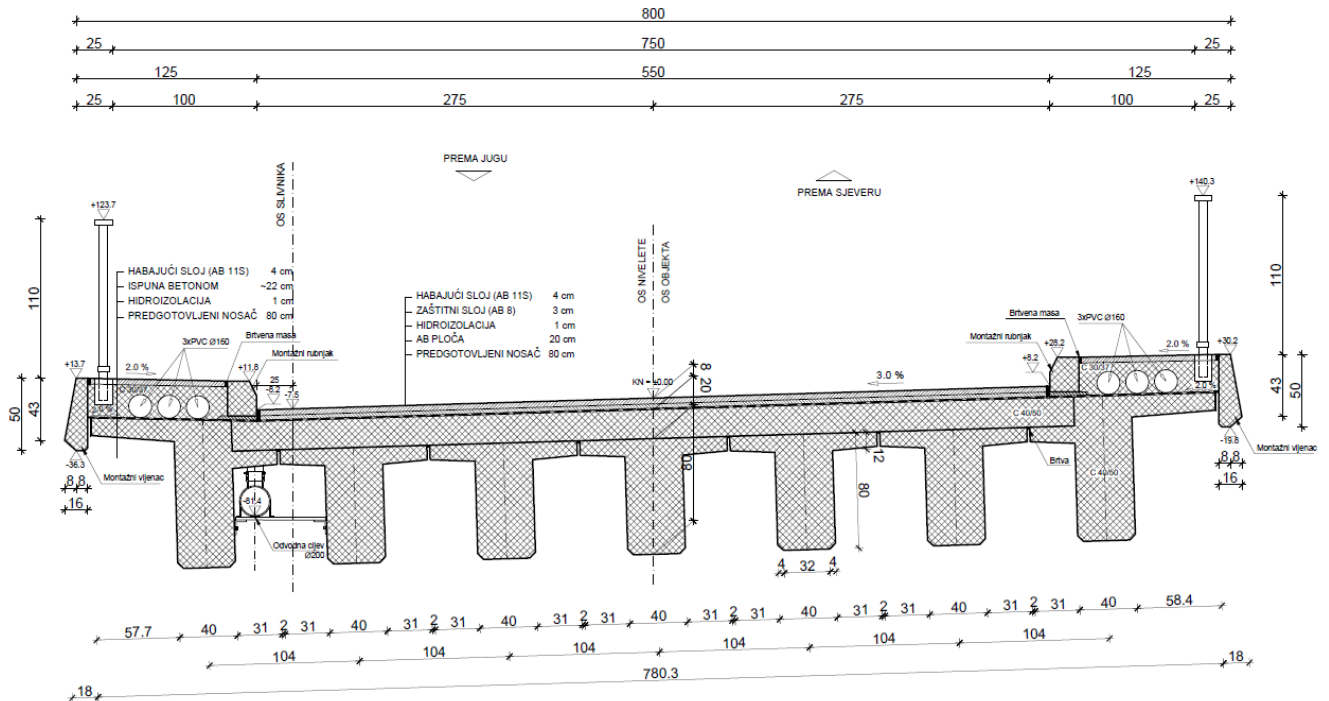
Slika 1: Poprečni presjek rasponske konstrukcije
