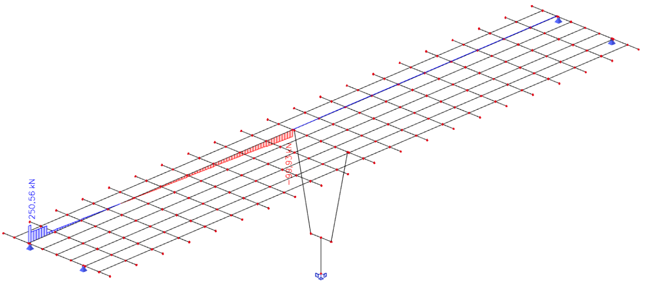
Slika 26: Pokretno opterećenje – maksimalna poprečna sila pri upornjaku – poprečne sile ( V_z ) u kN
