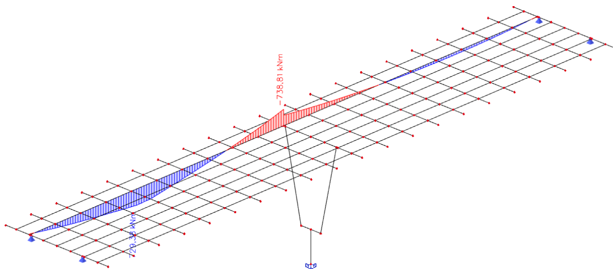
Slika 21: Pokretno opterećenje – maksimalni moment savijanja pri stupu – momenti savijanja ( M_y ) u kNm
