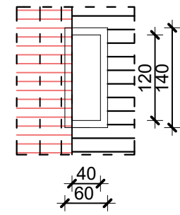
Tlocrt dimnjaka
