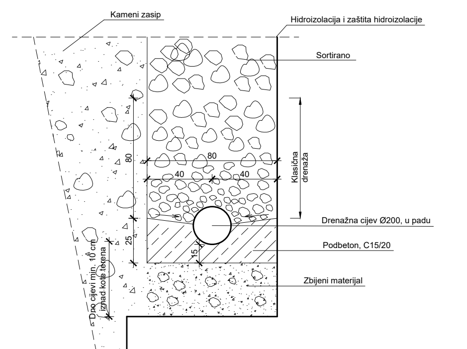
Detalj drenaže
