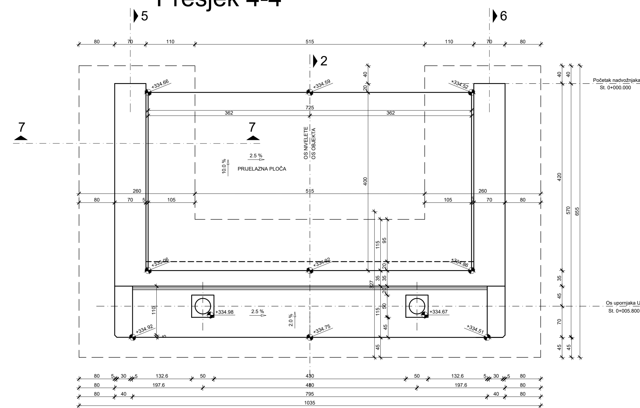
Presjek 4-4
