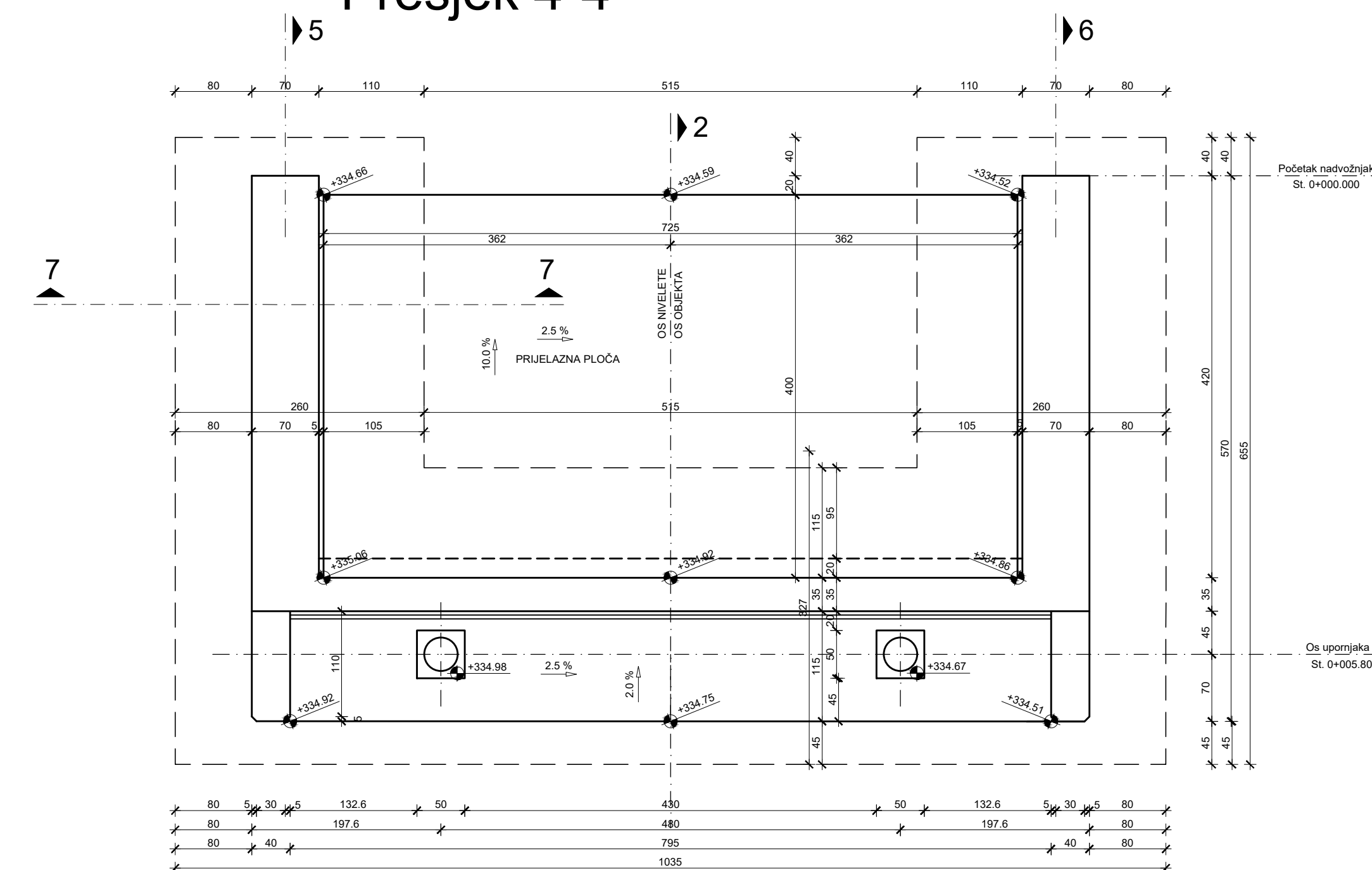
Presjek 4-4
