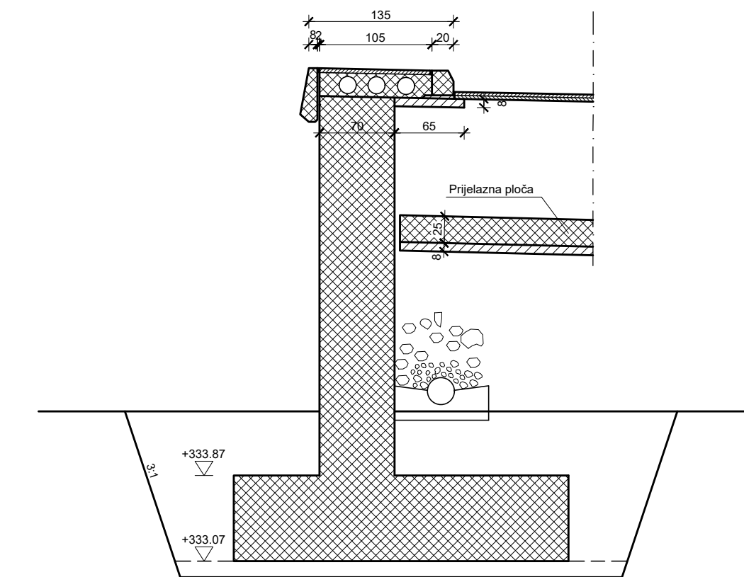
Presjek 7-7
