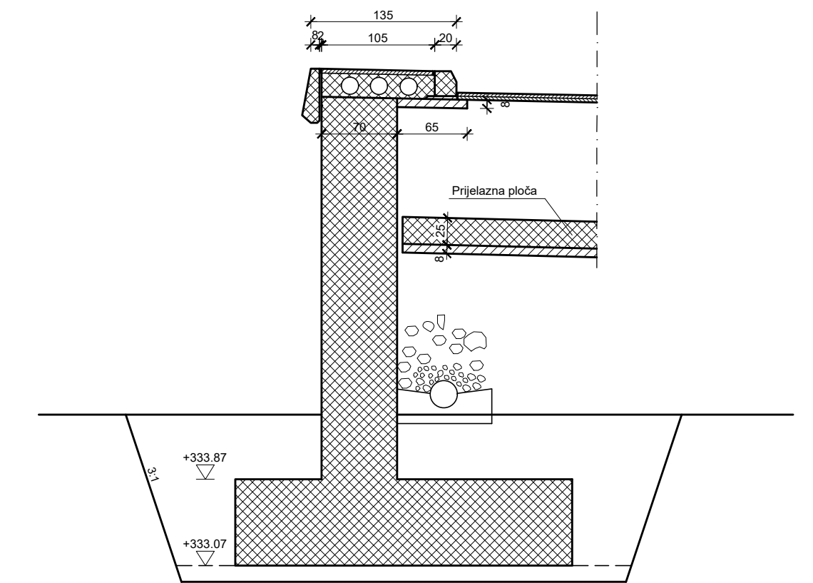
Presjek 7-7
