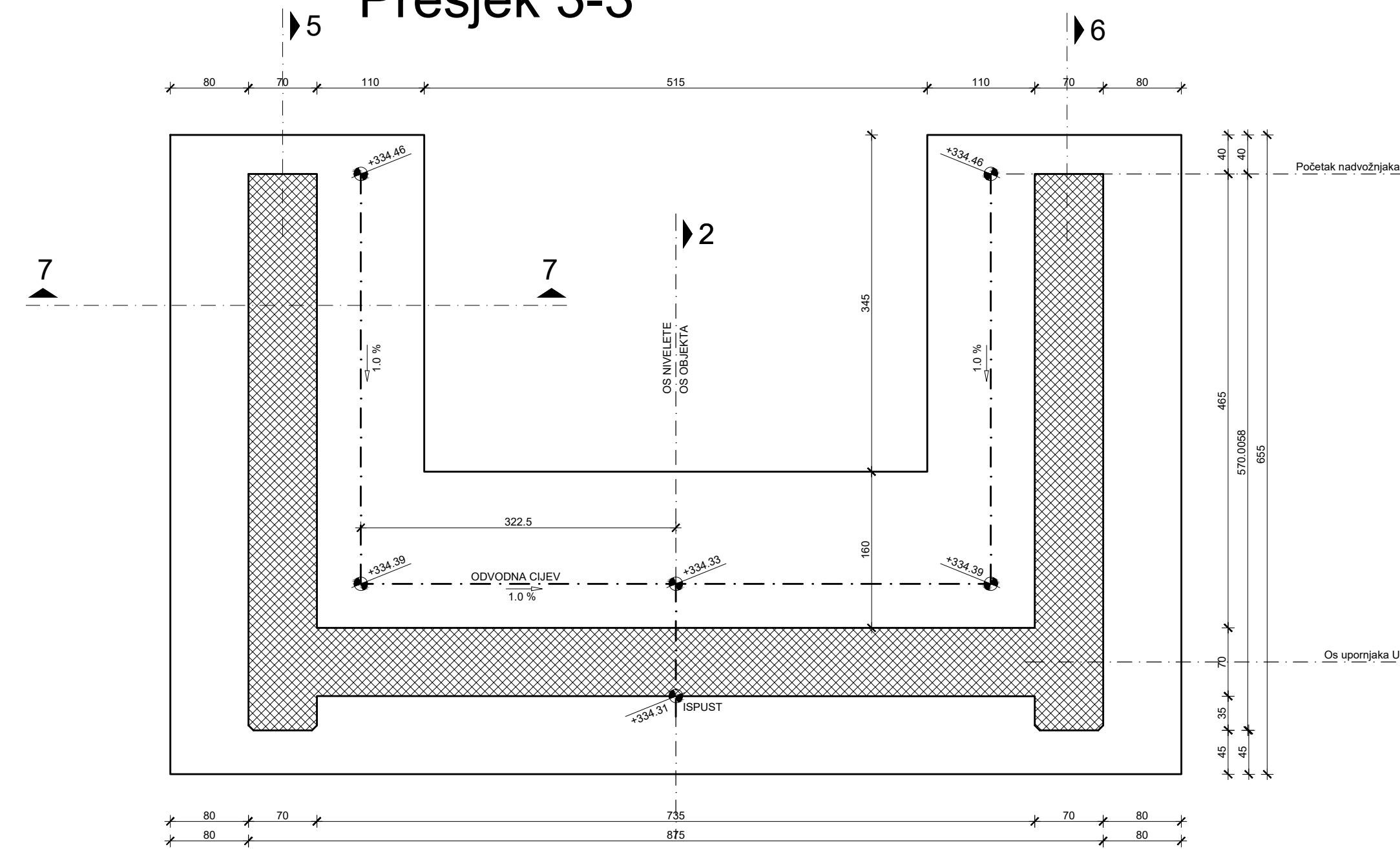
Presjek 3-3
