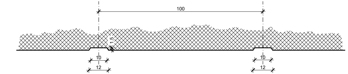
Detalj kanelura
