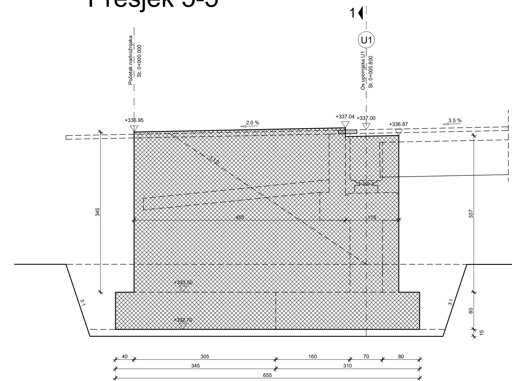
Presjek 5-5
