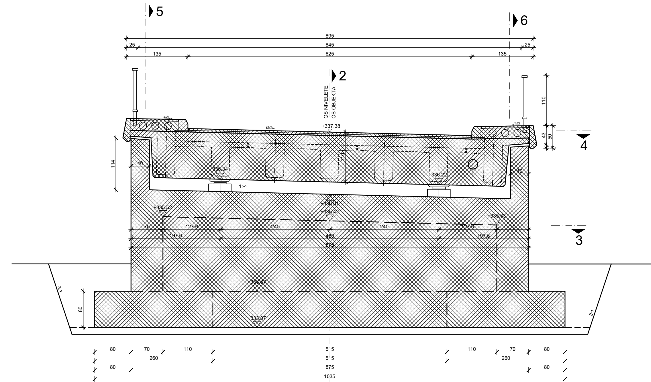
Presjek 1-1
