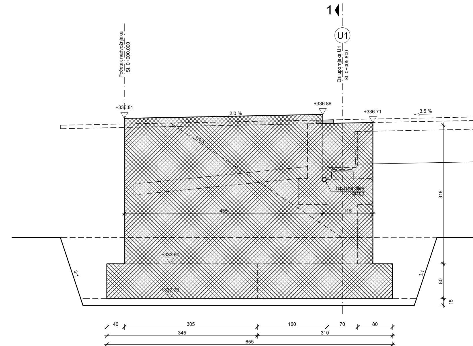
Presjek 6-6
