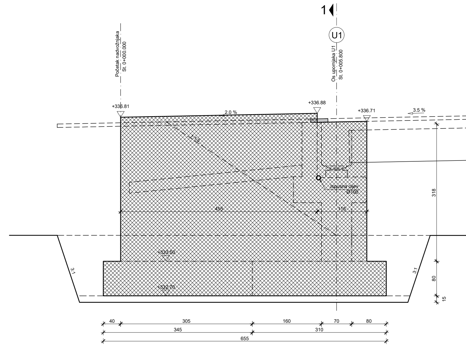
Presjek 6-6
