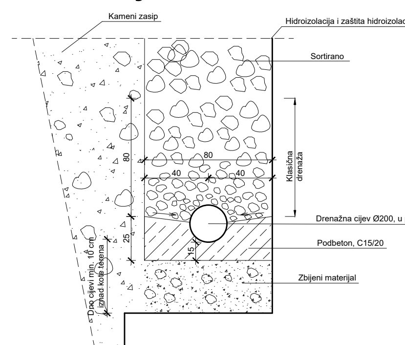
Detalj drenaže
