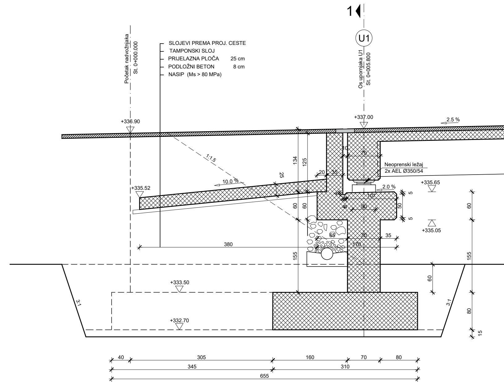
Presjek 4-4
