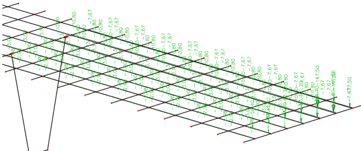
Slika 23: Pokretno opterećenje za maksimalnu poprečnu silu pri upornjaku
