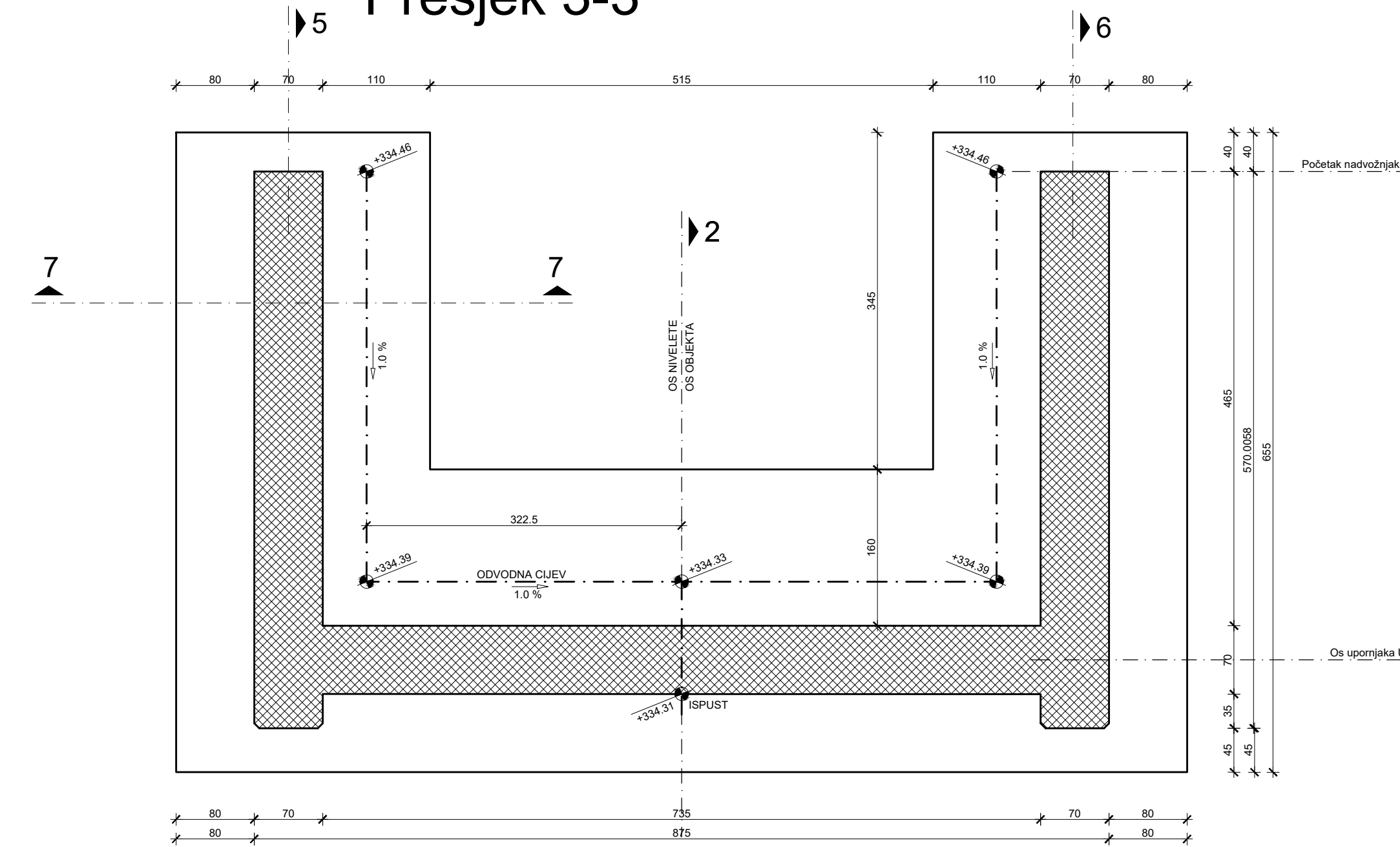
Presjek 3-3
