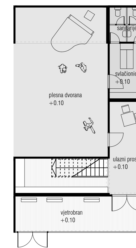
tlocrt prizemlja
