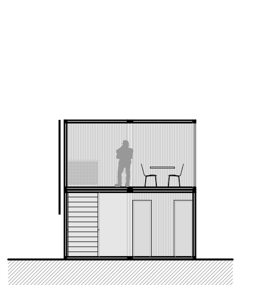
presjek
