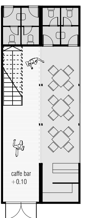
tlocrt prizemlja
