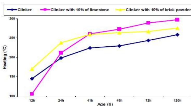
Slika 5.1: Utjecaj WCB na razvoj topline hidratacije[13]
