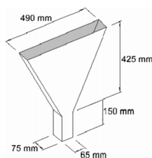
Slika 3.2: Dimenzije V-lijevka [7]
