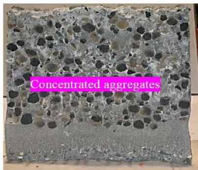
Slika 5.12: primjer segregacije po betonskom presjeku[17]
