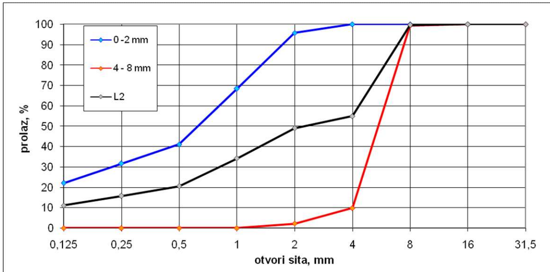
Slika 6.4: Granulometrijska krivulja za L2 mješavinu
