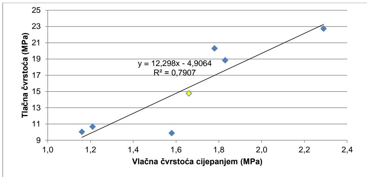
Slika 5.31 Veza između tlačne čvrstoće i vlačne čvrstoće cijepanjem
