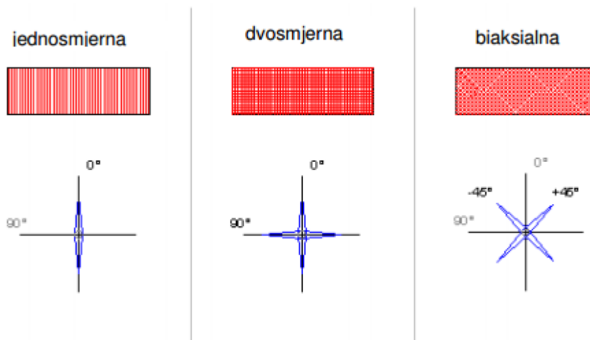
Crtež 2.5. Tipovi traka karbonskih vlakana i platna
