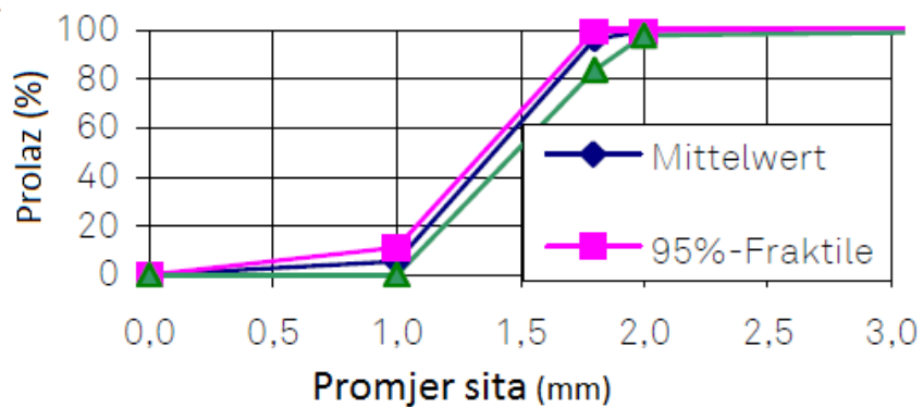
Slika 4.6. Granulometrijska krivulja Liaver ekspaniranoga stakla
