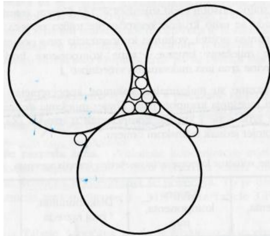
Slika 2.8. Interferencija zrna[8]
