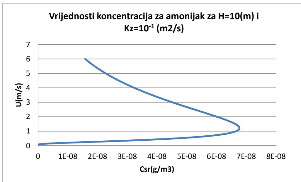
Slika 8.8. Srednje vrijednosti koncentracije po brzini za K_z=10^{-1} (m 2 /s) za sumporovodik i merkaptane za dimnjak visine 10(m)
