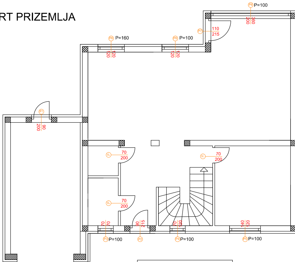
TLOCRT KATA
