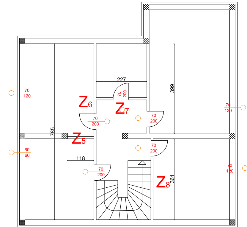
TLOCRT KATA
