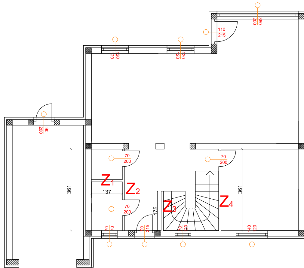
TLOCRT PRIZEMLJA
