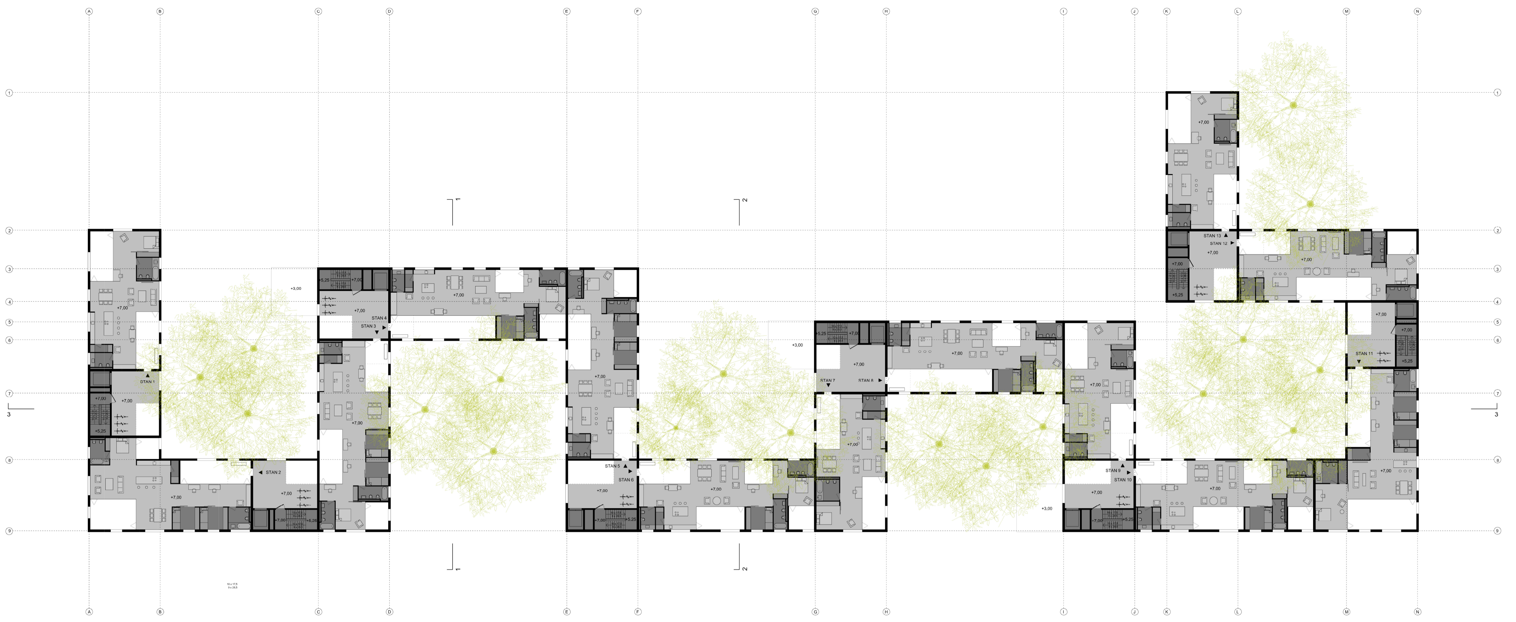
*tlocrt prve etaže +7,10
