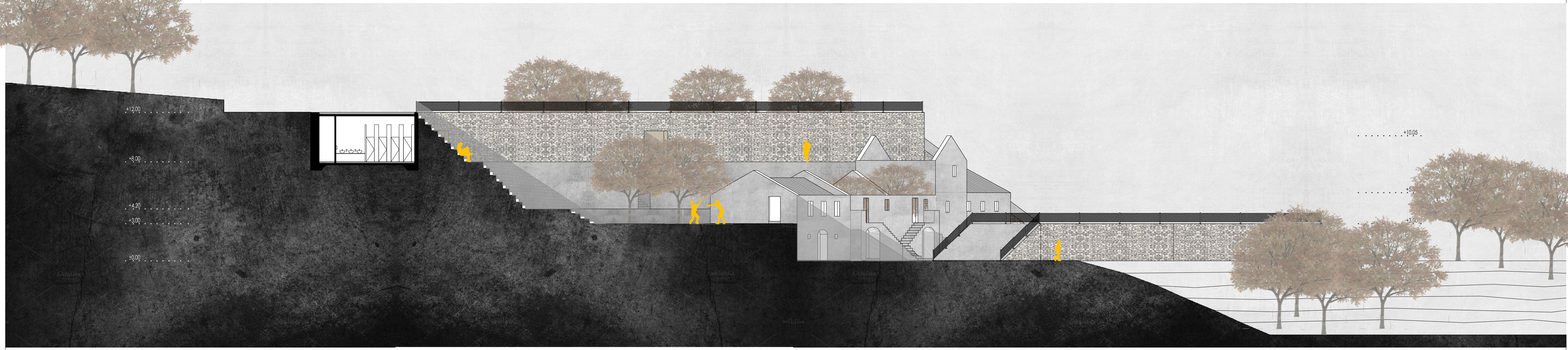
PRESJEK 3 - 3
