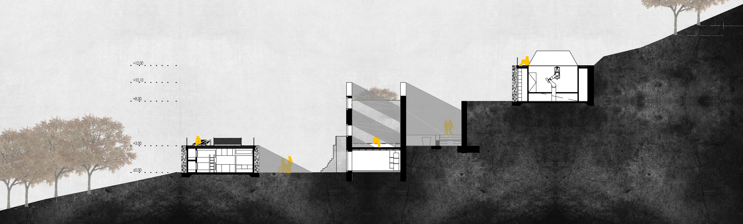
PRESJEK 2 - 2
