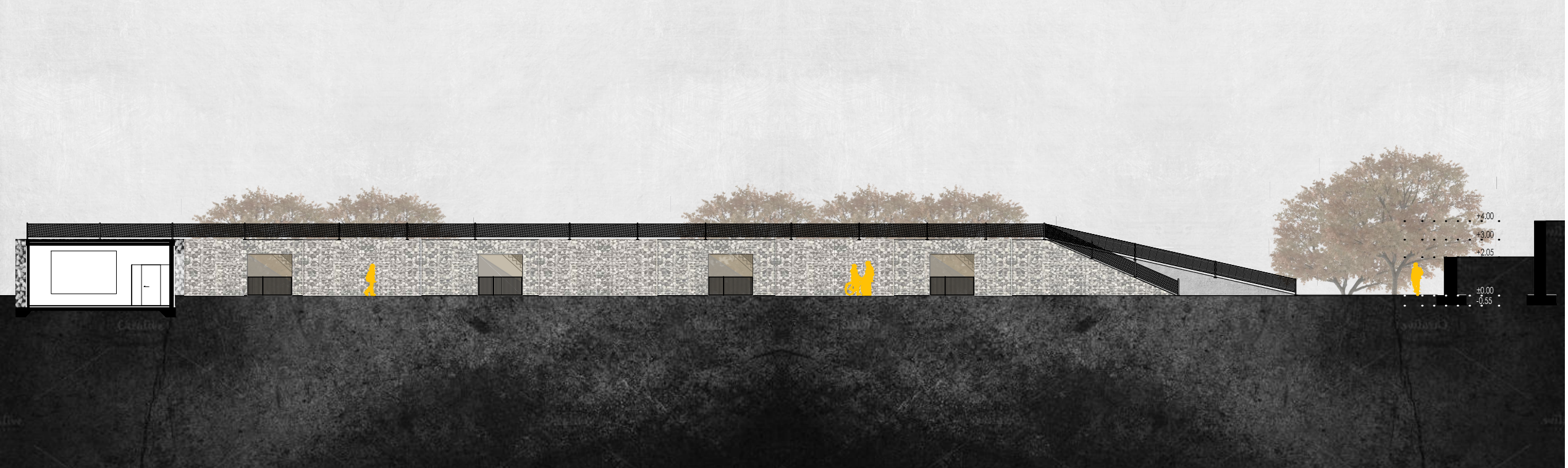
PRESJEK 4 - 4
