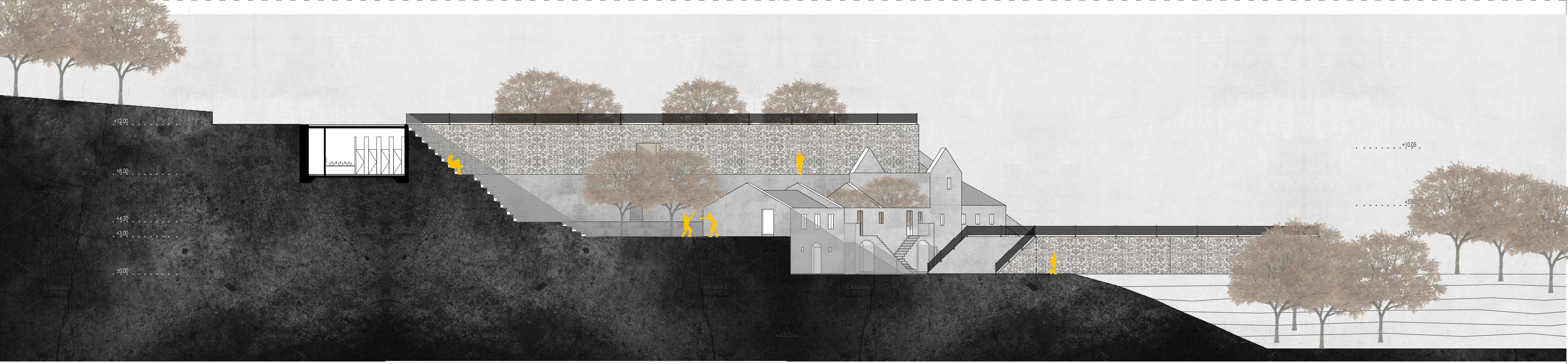
PRESJEK 3 - 3
