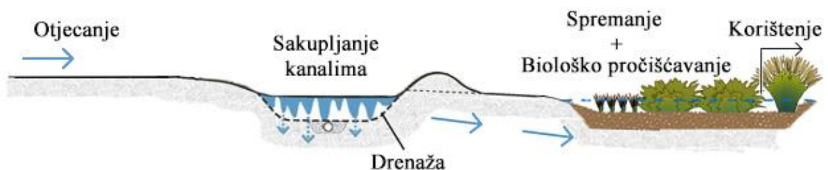
Slika 37. Shema uređaja za sakupljanje – spremanje + pročišćavanje
