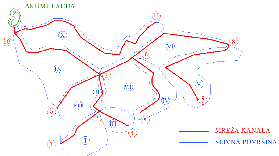
Slika 39. Shema oborinske mreže cijevi – akumulacija
