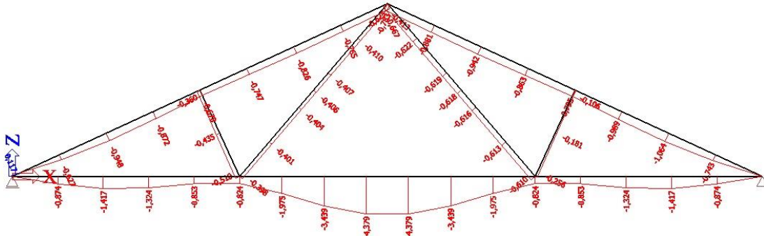
Slika 13. Prikaz progiba od vlastite težine G
