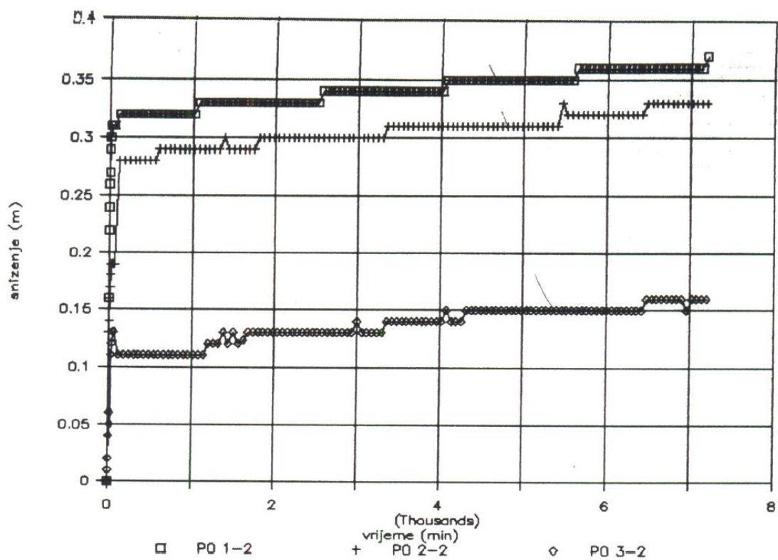
Slika 4.12 – Snižanja piezometara na dubini od 9,5 m
