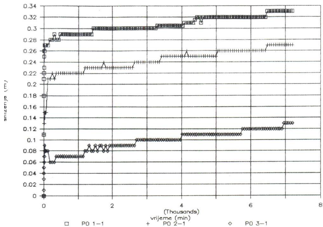
Slika 4.11 – Snižanja piezometara na dubini od 4,5 m
