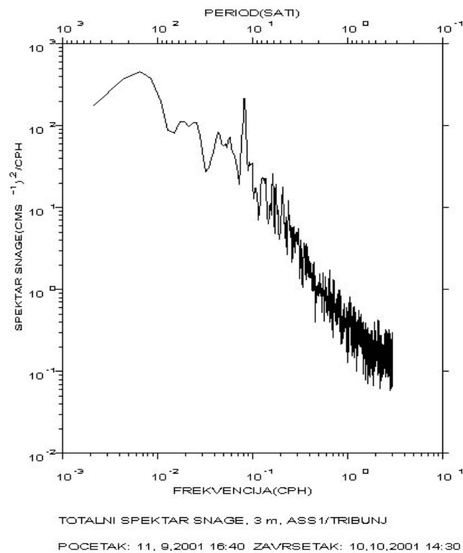
Slika 3.13. Totalni spektar snage morskih struja u pridnom sloju na postaji ASS-1 [2]
