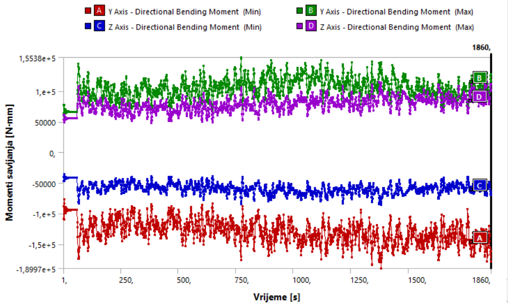
3.43 Max momenti savijanja u elementima
